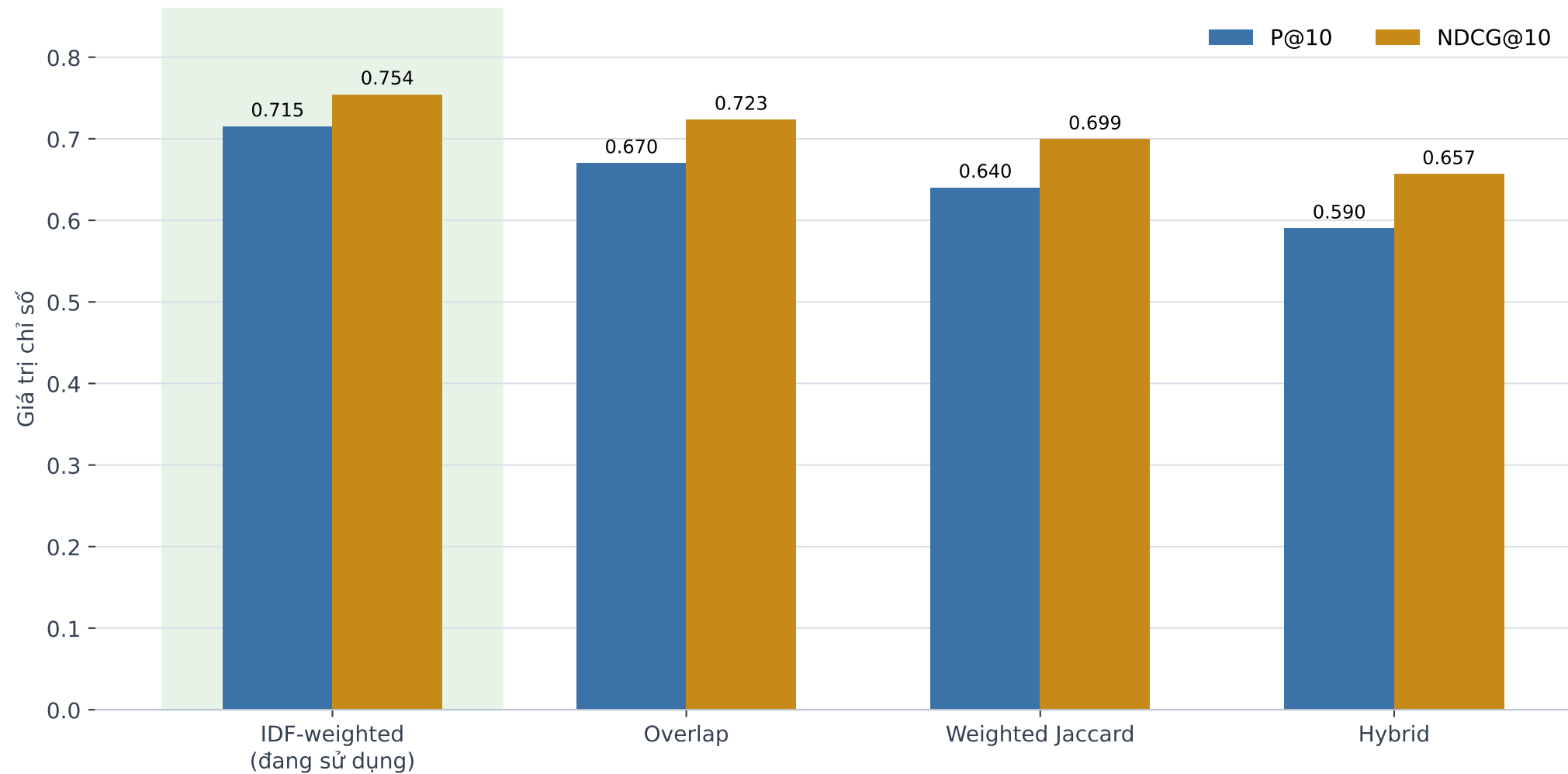
So sánh các phương pháp xếp hạng trên 20 trường hợp kiểm thử
