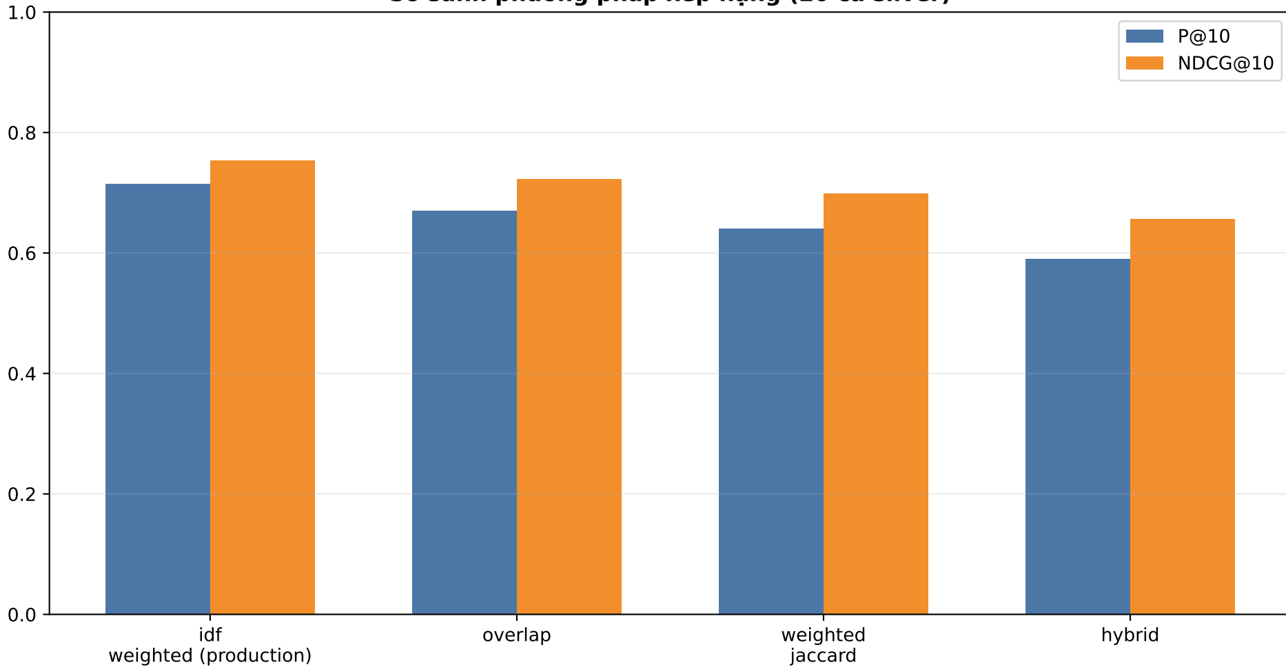
So sánh phương pháp xếp hạng (20 ca silver)
