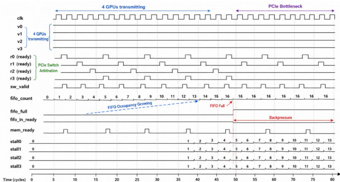
Hình 4.4. Timing Diagram
