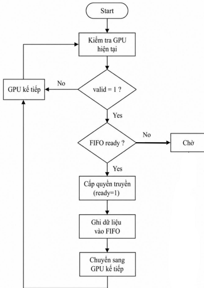
Hình 3.3: Lưu đồ Round-Robin của PCIe Switch
