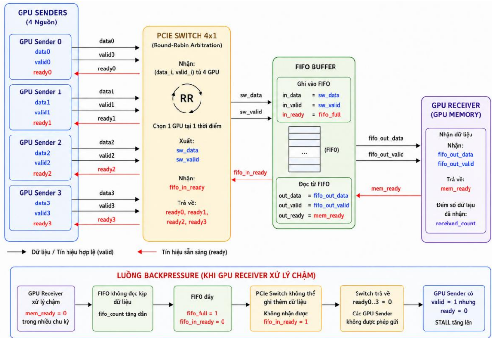
Hình 3.6: Sơ đồ protocol giữa các khối trong mô hình PCIe Intra-GPU Interconnect
