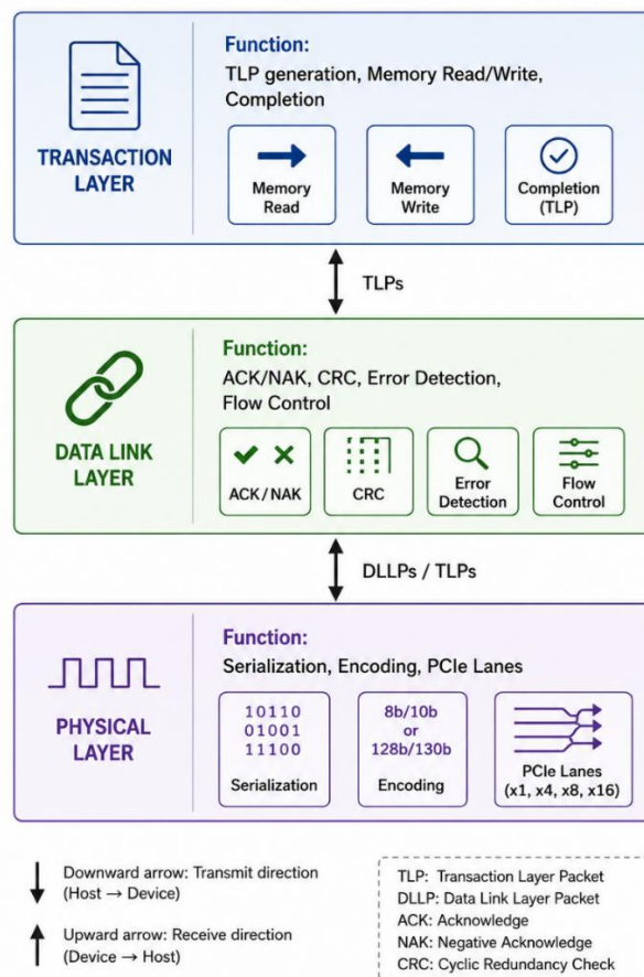
Hình 2.8: Kiến trúc giao thức PCIe
