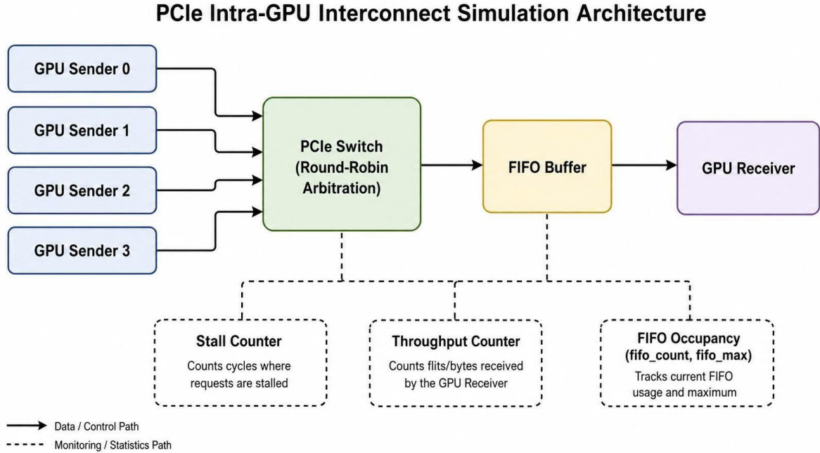
Hình 3.1. Sơ đồ khối tổng thể của mô hình PCIe Intra-GPU Interconnect
