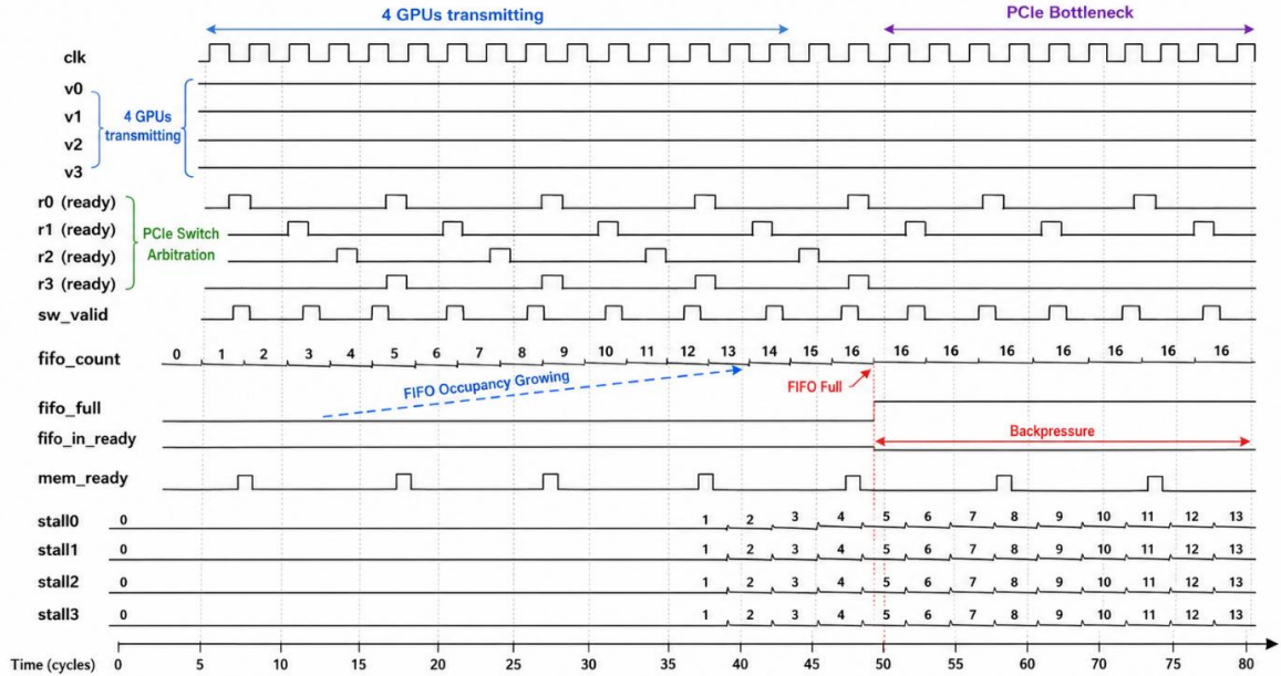
Hình 4.4. Timing Diagram
