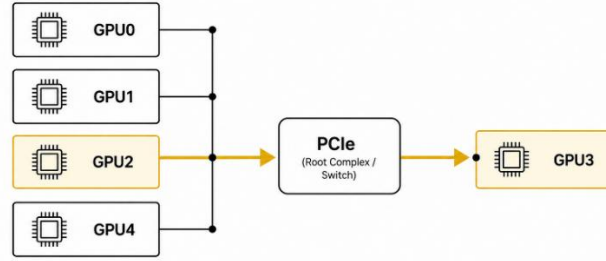
Hình ảnh 2.10: Ví dụ minh họa về việc trao đổi dữ liệu GPU
