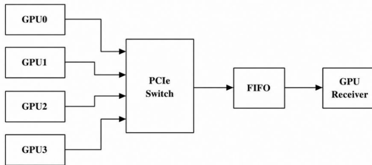
Hình ảnh 2.12: Bottleneck của PCIe
