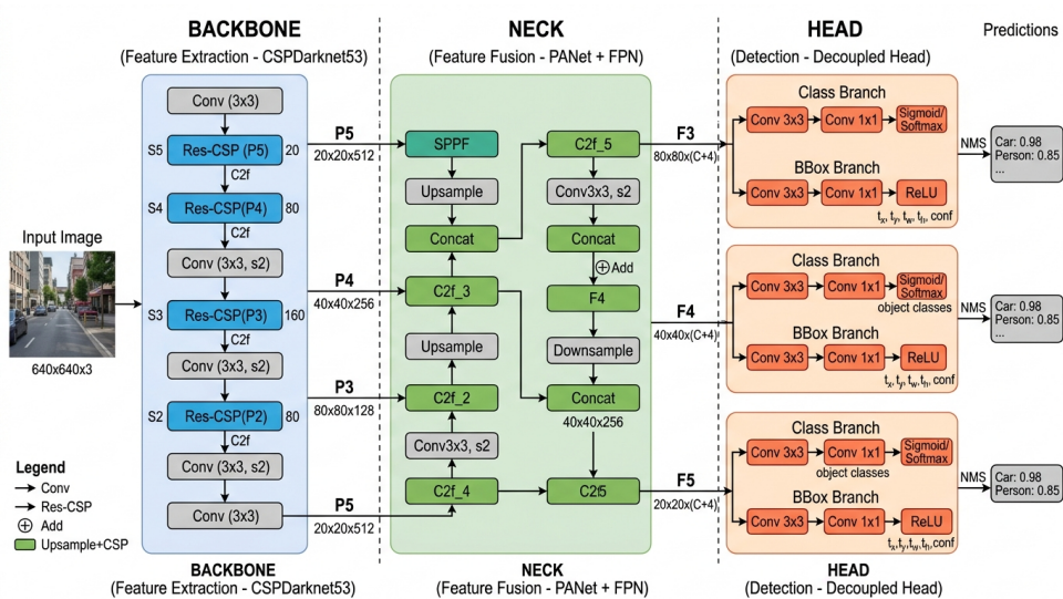
Hình 2.2: Cấu trúc khái quát của một detector YOLO gồm backbone, neck và head.
