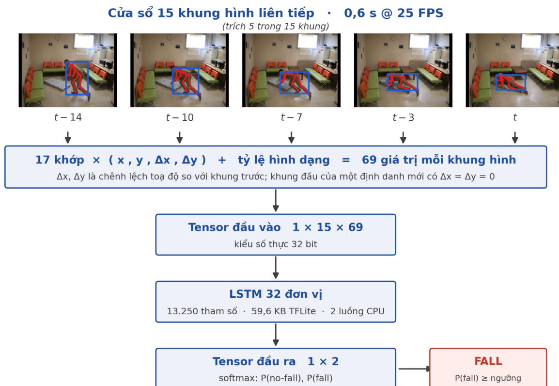
Hình 4.5: Chuỗi suy luận của khối LSTM phát hiện té ngã. Năm khung hình được trích từ cửa sổ 15 khung của video Coffee_room_01 , kèm khung xương 17 điểm và hộp bao do YOLO26n-Pose sinh ra.
