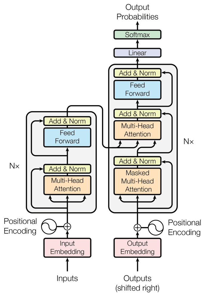
Hình 2.7: Sơ đồ kiến trúc của mô hình Transformer với cơ chế Multi-Head Attention.
