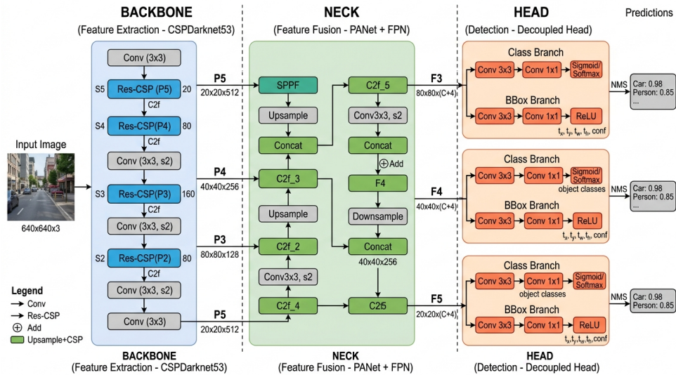
Hình 2.4: Minh họa một kiến trúc mạng YOLO tiêu biểu với Backbone, Neck và Head.
