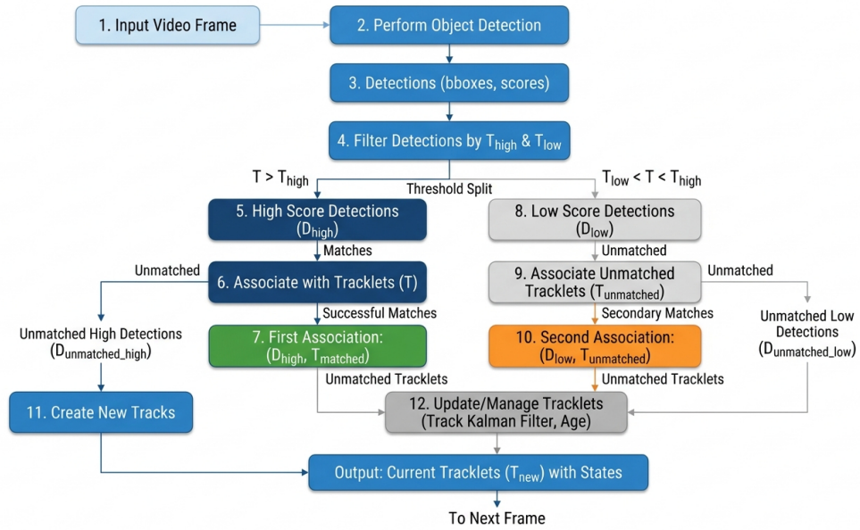
Hình 2.5: Thuật toán ByteTrack với cơ chế Dual-threshold Association giúp duy trì Track ID ổn định.
