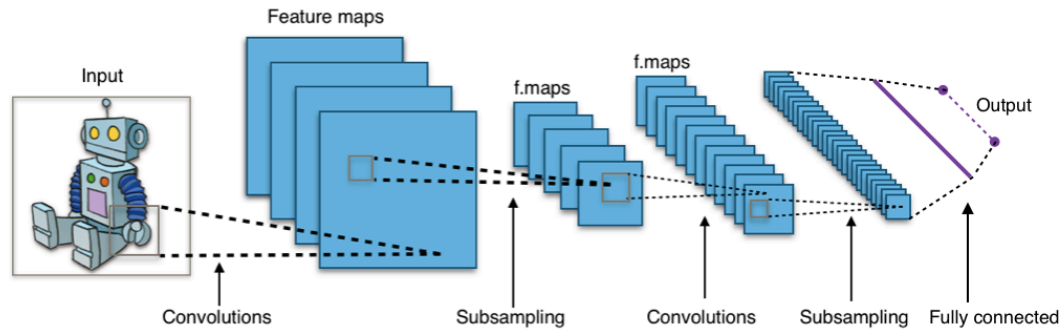
Hình 2.3: Minh họa cấu trúc tiêu biểu của mạng nơ-ron tích chập (CNN) gồm các lớp Convolution, Pooling và Fully Connected.
