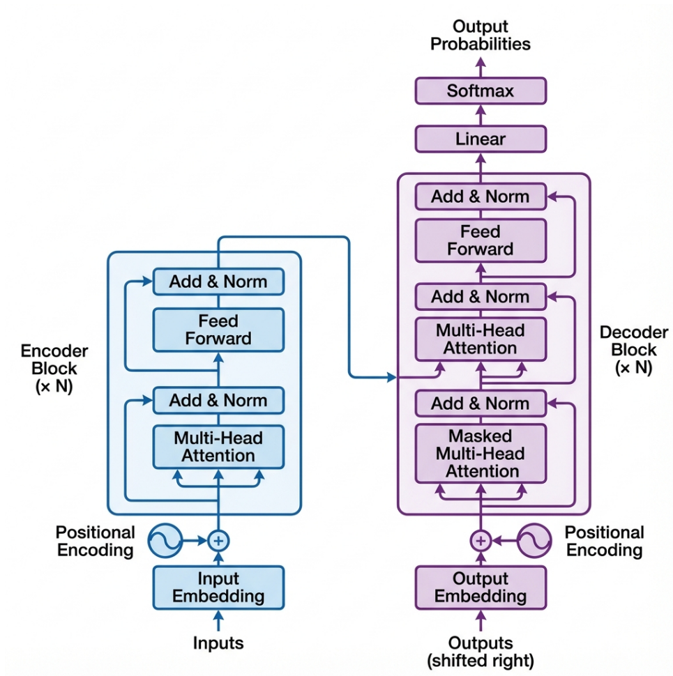
Hình 2.9: Kiến trúc Transformer với các khối Encoder và Decoder
