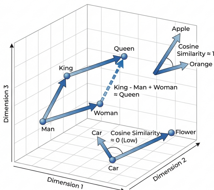
Hình 2.8: Minh họa không gian vector embedding và độ tương đồng cosine giữa các từ
