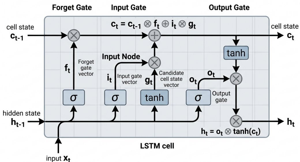
Hình 2.6: Cấu trúc chi tiết của một tế bào LSTM (LSTM cell) với hệ thống các cổng kiểm soát thông tin.
