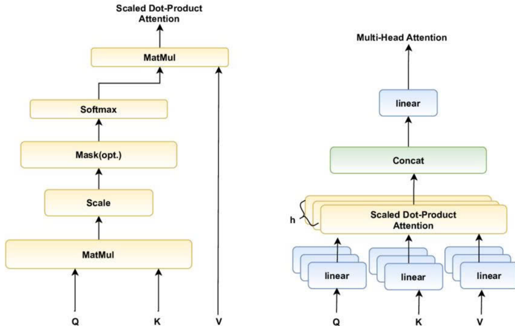
Hình 2.10: Cơ chế Self-Attention: Query, Key, Value và Scaled Dot-Product Attention
