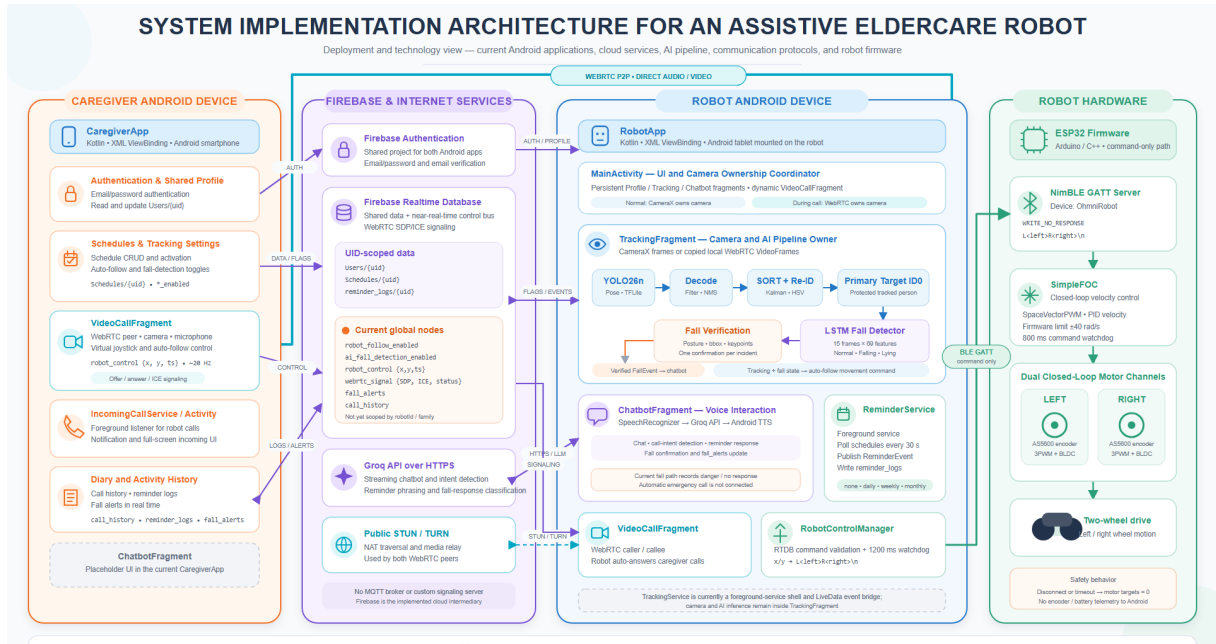
Hình 3.5: Kiến trúc hiện thực của hệ thống
