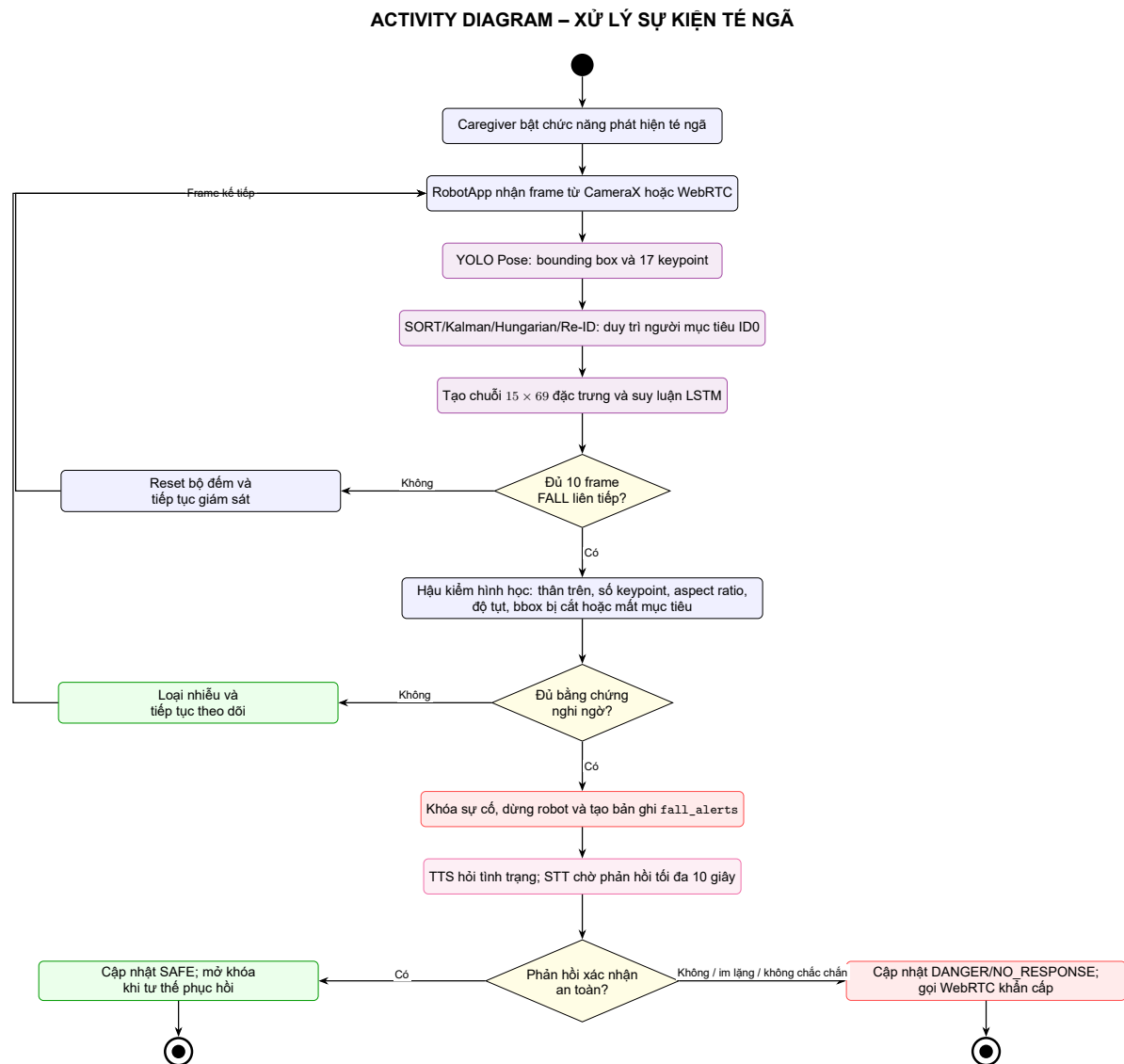
Hình 3.3: Biểu đồ hoạt động của quy trình phát hiện, hậu kiểm và xử lý té ngã
