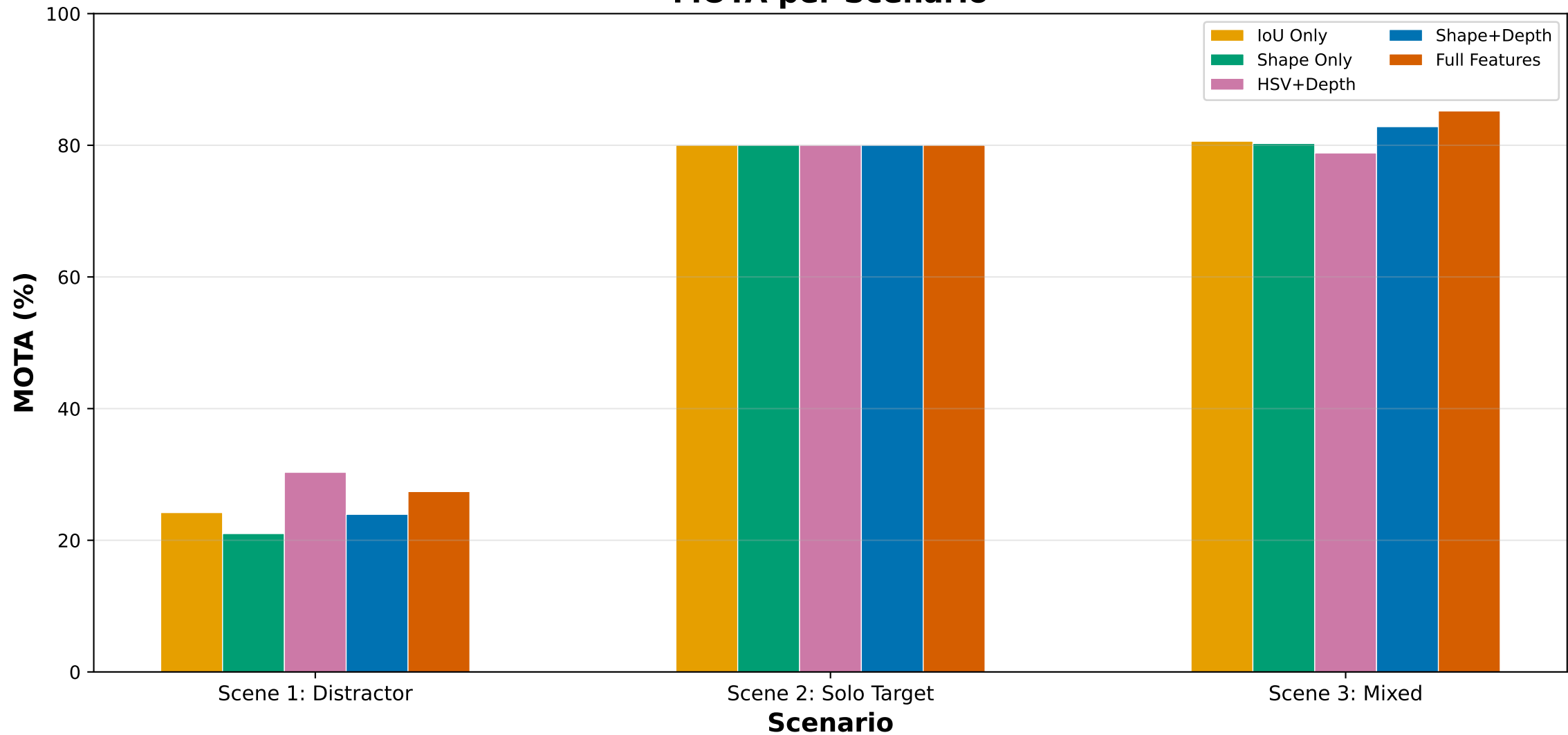
MOTA per Scenario
