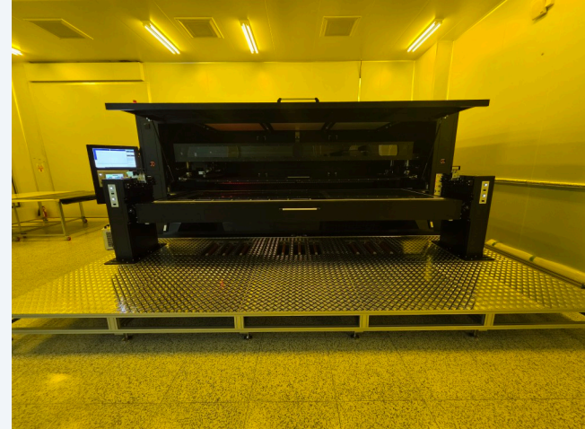
ACC Support Stick용 8.7G LED 노광기 / 원본 제시 설비
