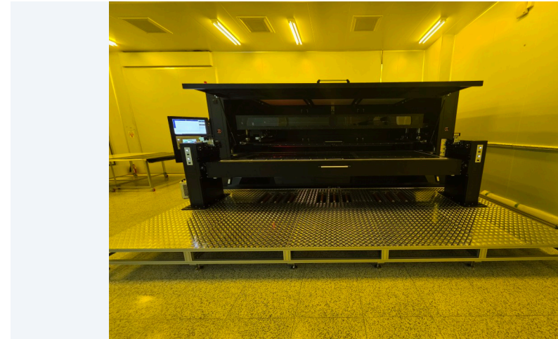
ACC Support Stick용 8.7G LED 노광기 / 원본 제시 설비
