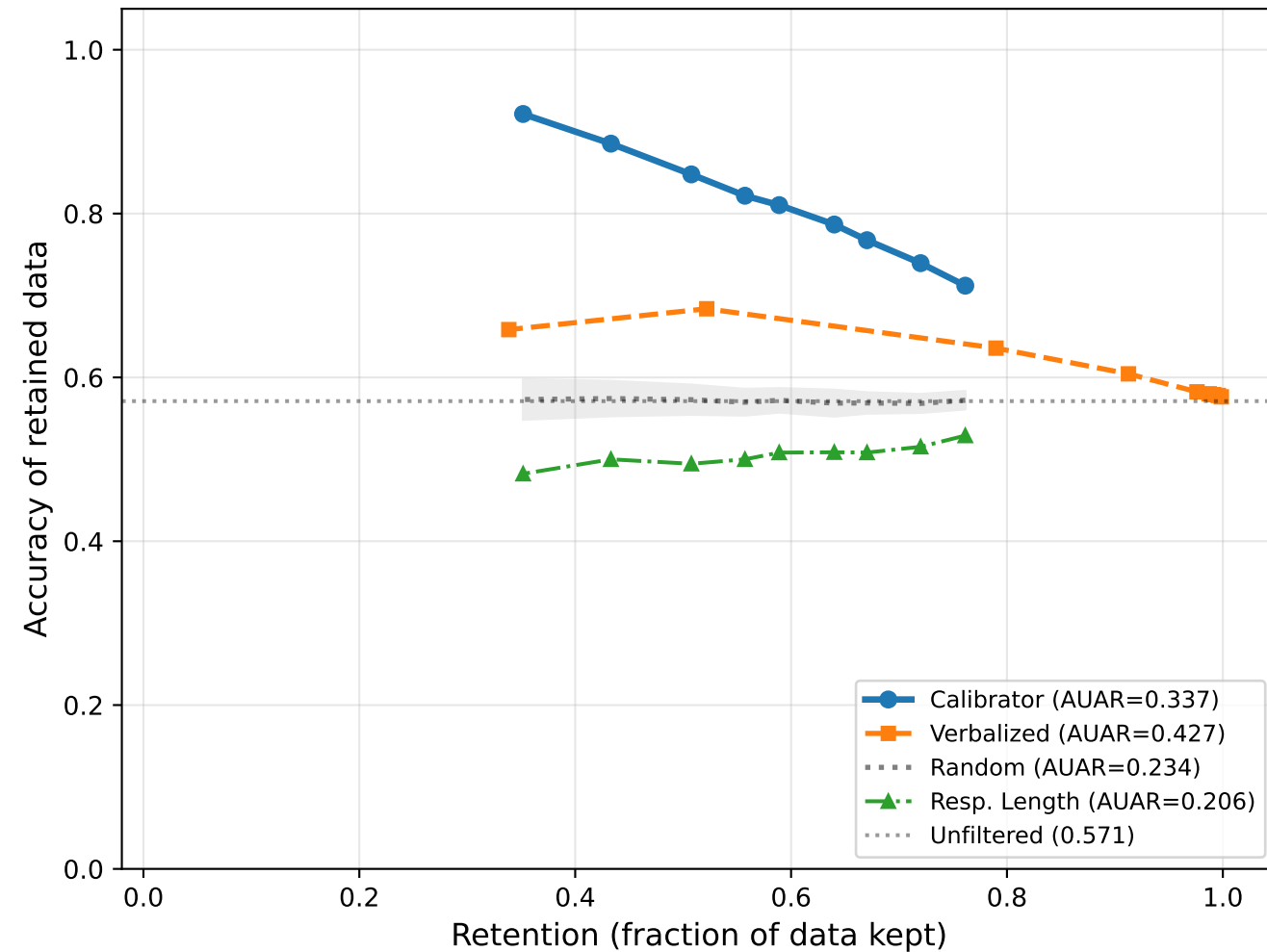
GPT-5.2 (N=725)
