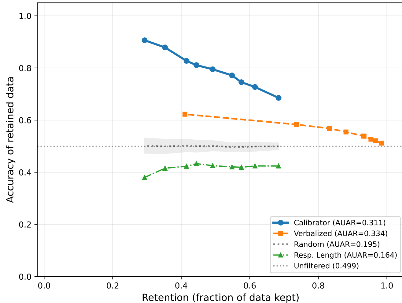
GPT-5-mini (N=655)
