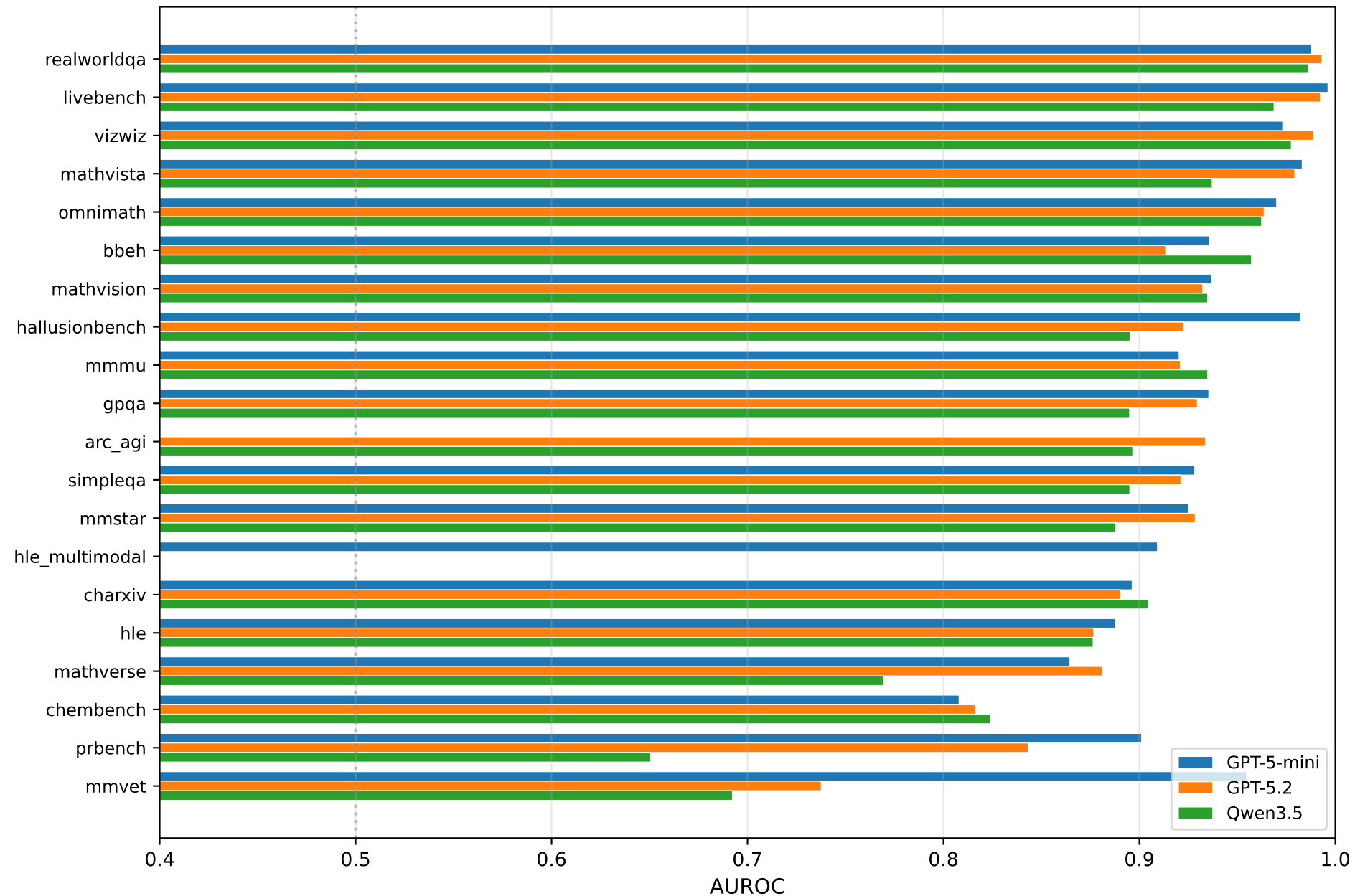
Per-Benchmark Calibrator AUROC
