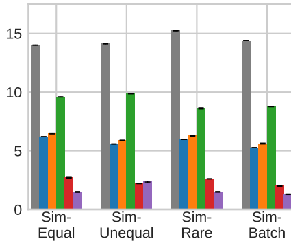
Dropout-MSE
