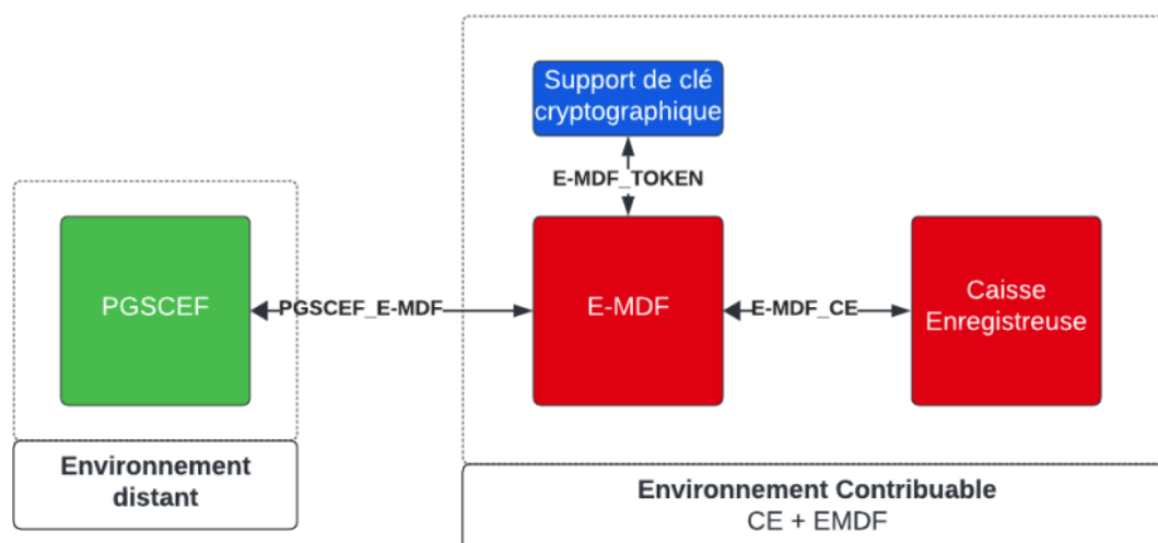
Figure 1 : Architecture du système de caisses enregistreuses fiscales (SCEF)
