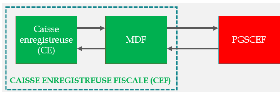
Figure 1 : Architecture du système de caisses enregistreuses fiscales.
