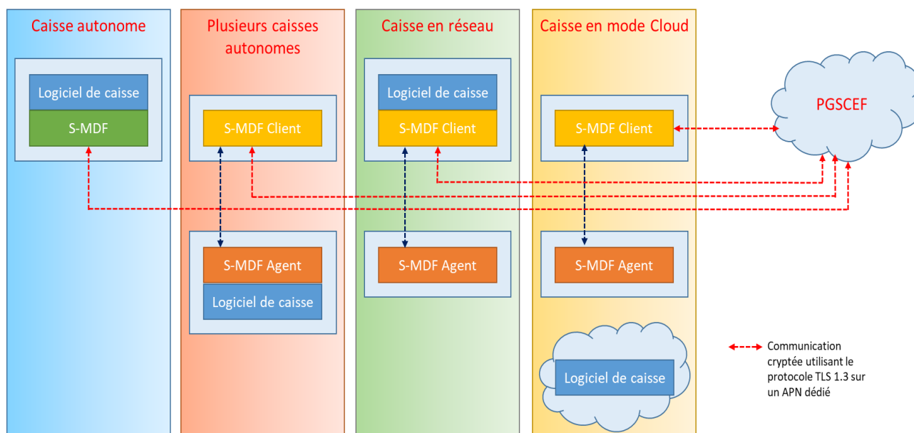
Figure 3 : Modes de déploiement des S-MDF.
