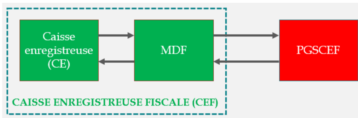
Figure 2 : Architecture du système de caisses enregistreuses fiscales.
