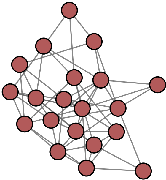
(a) Erdős-Rényi
