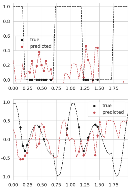
P-VAE
