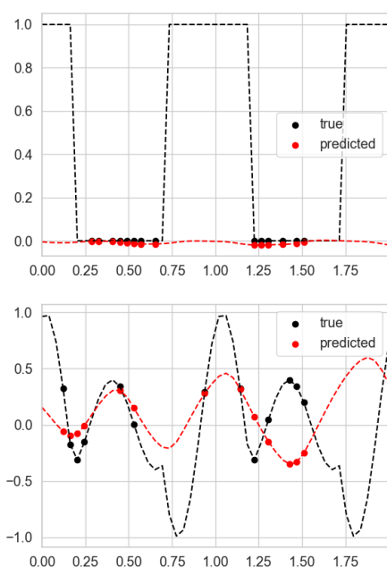
Latent ODE
