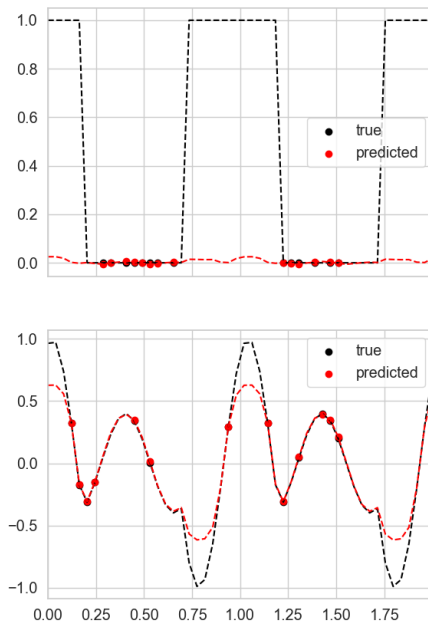
Latent ODE
