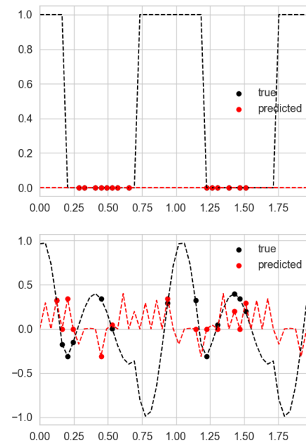
LLMTime
