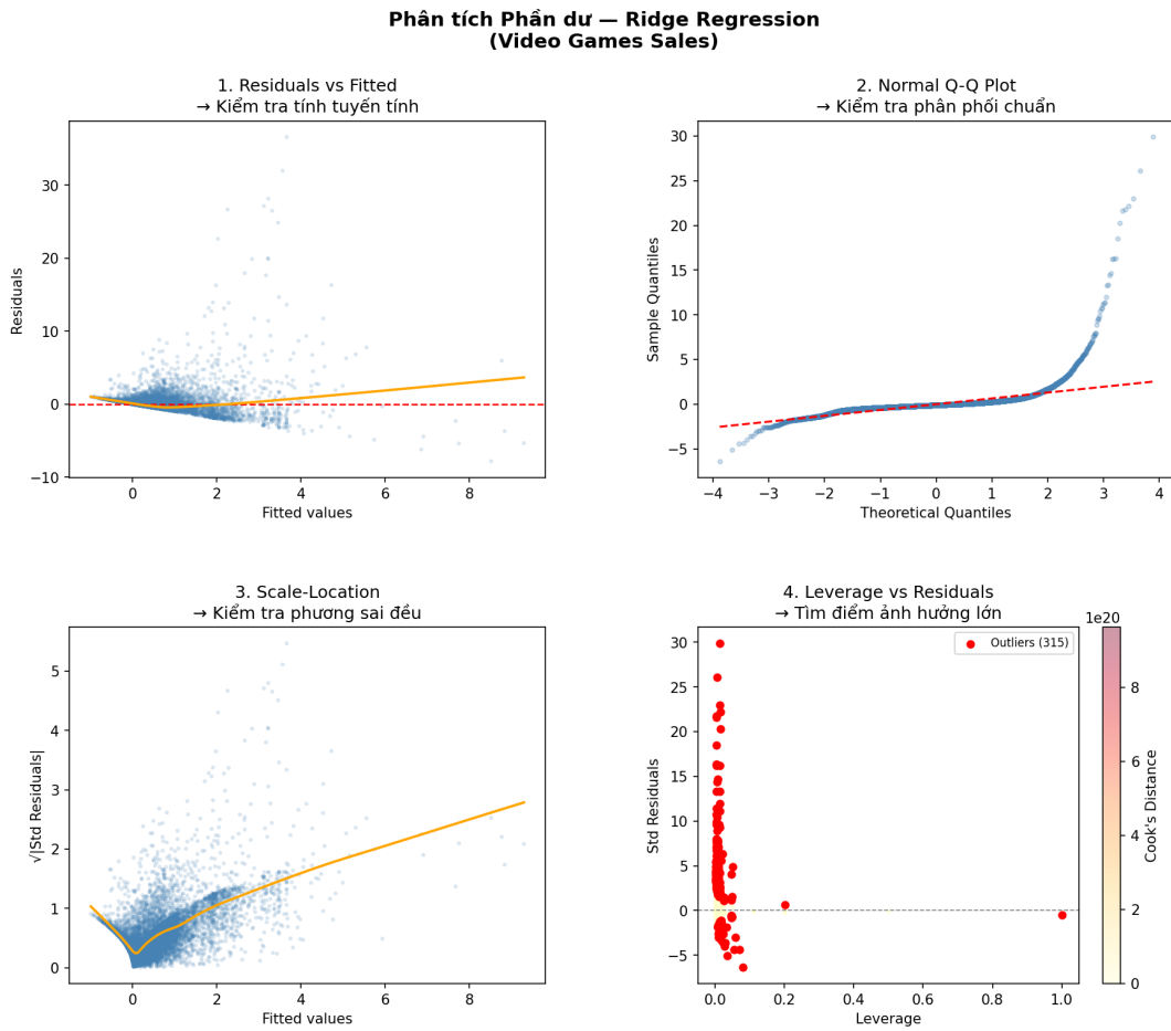
Hình 7: Biểu đồ chẩn đoán phần dư của mô hình Ridge Regression.
