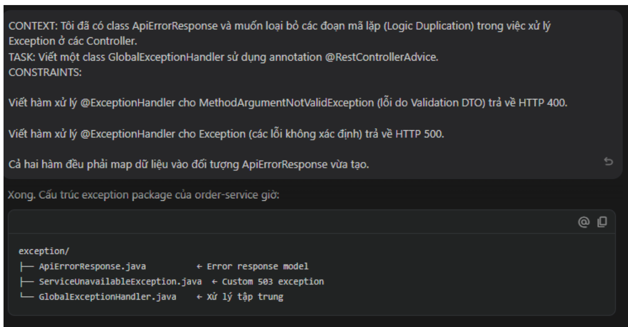
Hình 15: Prompt tạo Global Exception Handler và các định dạng JSON lỗi đồng nhất (p1)
