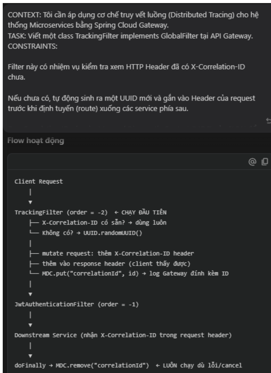
Hình 28: : Prompt yêu cầu tạo TrackingFilter và sơ đồ luồng hoạt động do AI phác thảo
