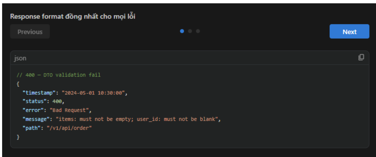
Hình 16: Prompt tạo Global Exception Handler và các định dạng JSON lỗi đồng nhất (p2)
