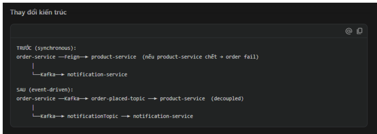
Hình 7: Tái cấu trúc logic lỗi (Refactoring OrderService) (p3)
