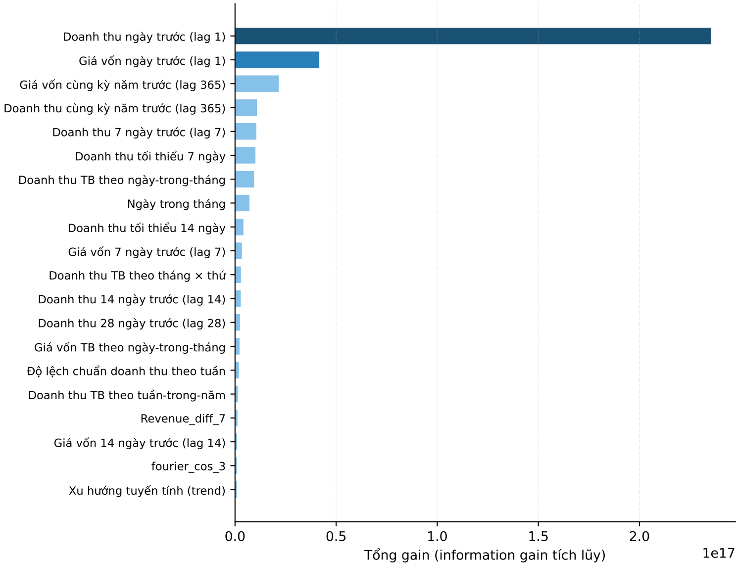
Top 20 đặc trưng theo LightGBM gain — mô hình doanh thu
