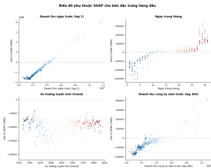
Figure 17: Biểu đồ phụ thuộc SHAP cho bốn đặc trưng hàng đầu. Trục hoành: giá trị gốc của đặc trưng; trục tung: giá trị SHAP (VND); màu sắc mã hóa giá trị đặc trưng. Đường nét đứt đánh dấu mức tác động bằng không.
