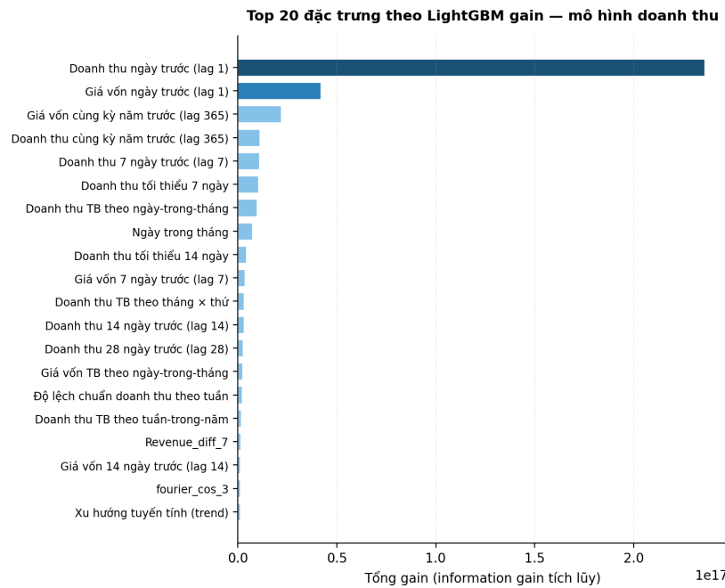
Figure 15: Top 20 đặc trưng theo tổng information gain tích lũy từ cấu trúc cây LightGBM. Cường độ màu tỷ lệ với mức đóng góp tương đối so với đặc trưng hàng đầu.
