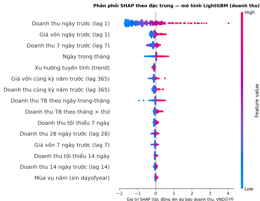
Figure 16: Biểu đồ beeswarm SHAP cho 15 đặc trưng hàng đầu. Mỗi điểm là một mẫu quan sát; trục hoành là giá trị SHAP (VND); màu sắc mã hóa giá trị gốc của đặc trưng (đỏ = cao, xanh = thấp).
