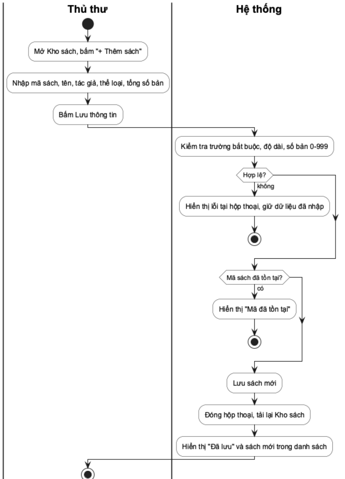
Hình 3.6. Sơ đồ hoạt động UC02 Thêm sách
