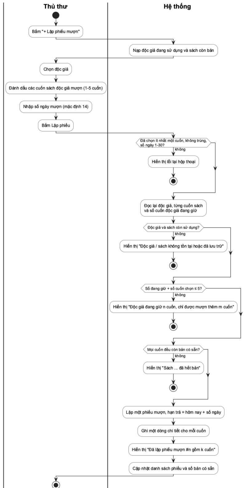
Hình 3.7. Sơ đồ hoạt động UC10 Lập phiếu mượn
