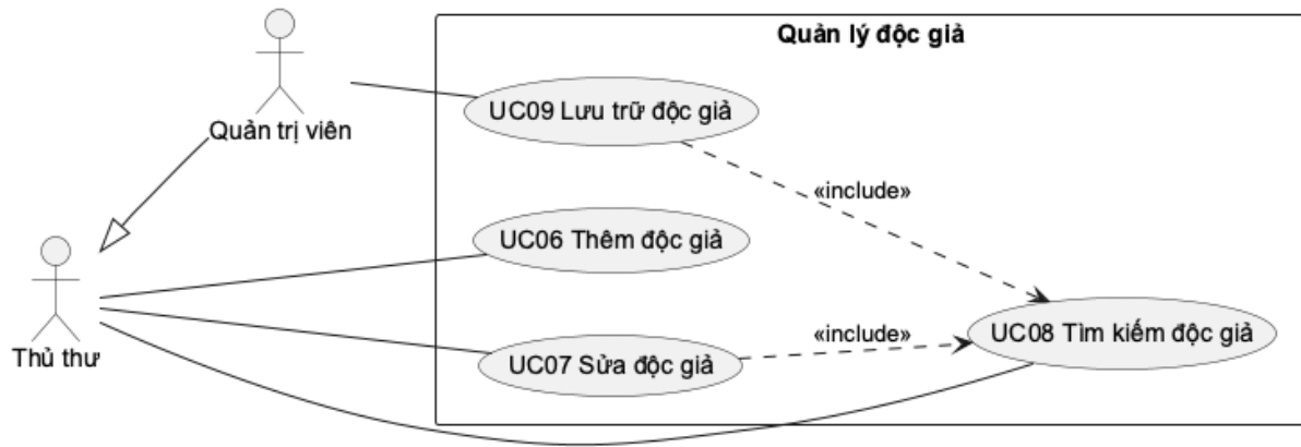
Hình 3.3. Phân rã use case Quản lý độc giả
