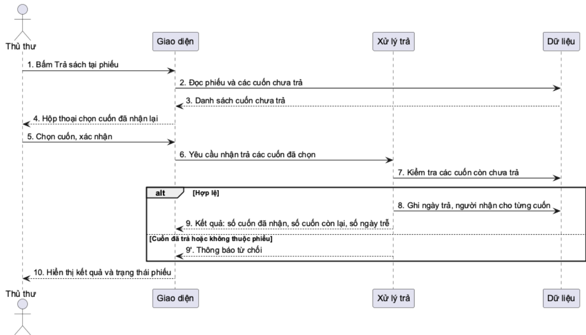
Hình 3.19. Sơ đồ tuần tự trả sách
