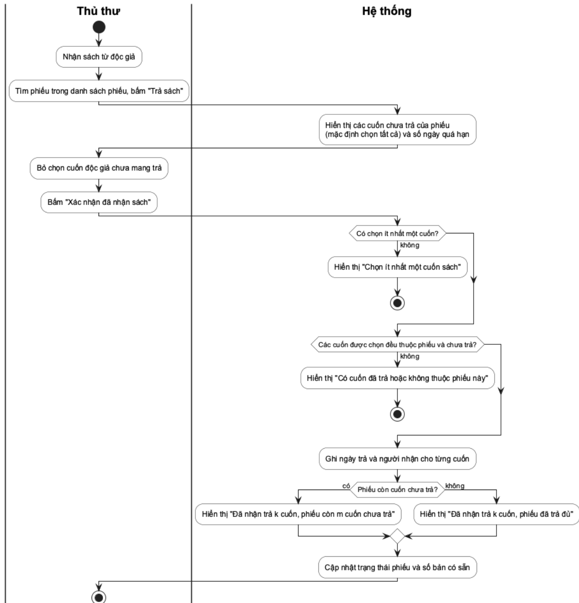
Hình 3.8. Sơ đồ hoạt động UC12 Trả sách
