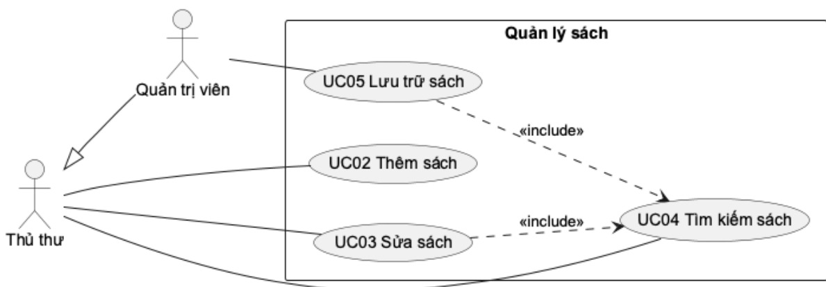
Hình 3.2. Phân rã use case Quản lý sách
