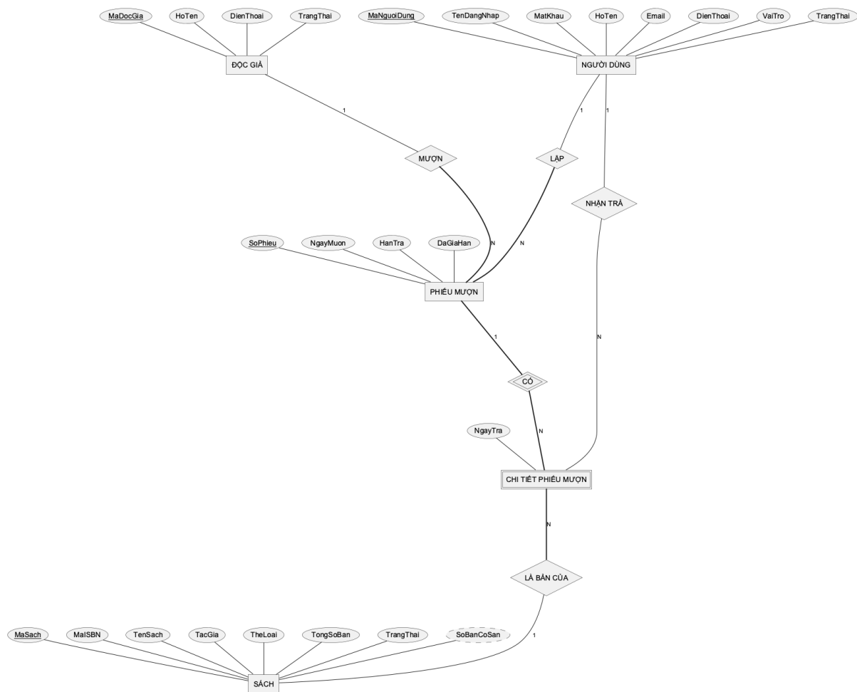
Hình 3.9. Mô hình ERD (kỹ pháp Chen)
