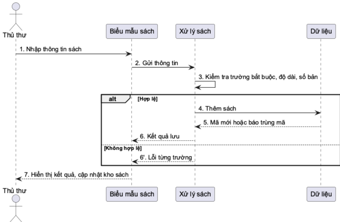
Hình 3.20. Sơ đồ tuần tự thêm sách
