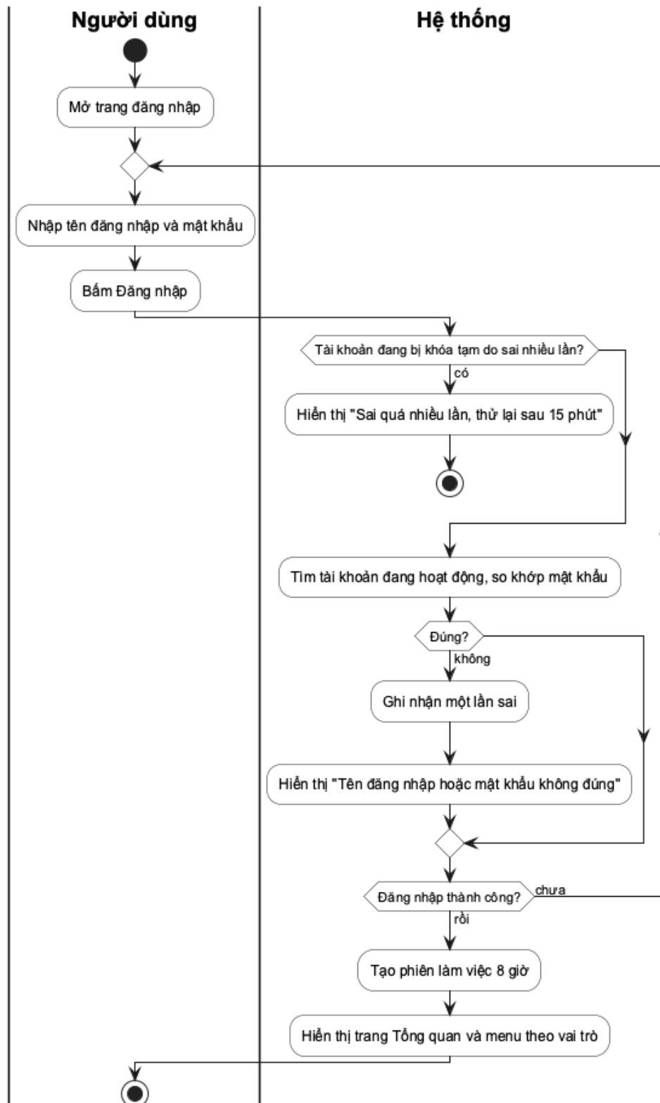
Hình 3.5. Sơ đồ hoạt động UC01 Đăng nhập
