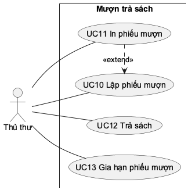
Hình 3.4. Phân rã use case Mượn trả sách
