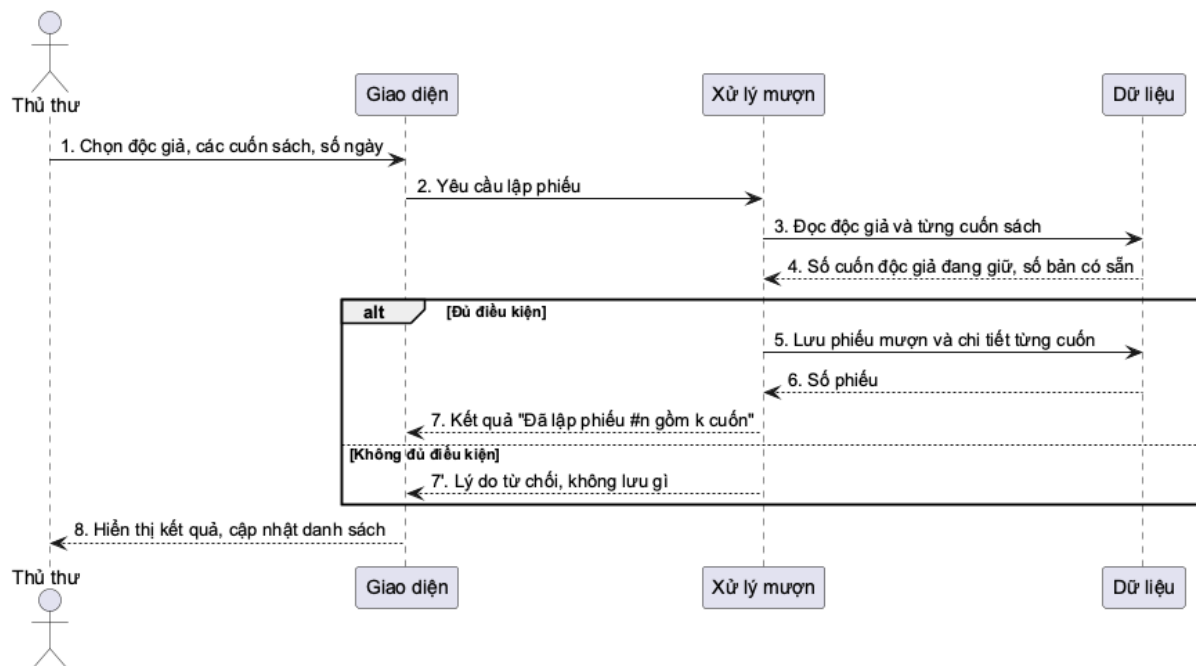
Hình 3.18. Sơ đồ tuần tự lập phiếu mượn
