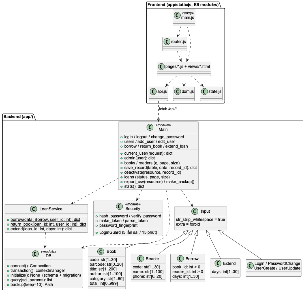
Hình 6. Module, DTO và LoanService thực tế
