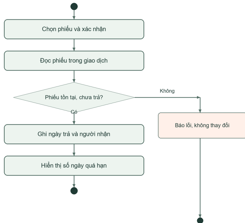
Hình 9. Luồng điều khiển trả sách
