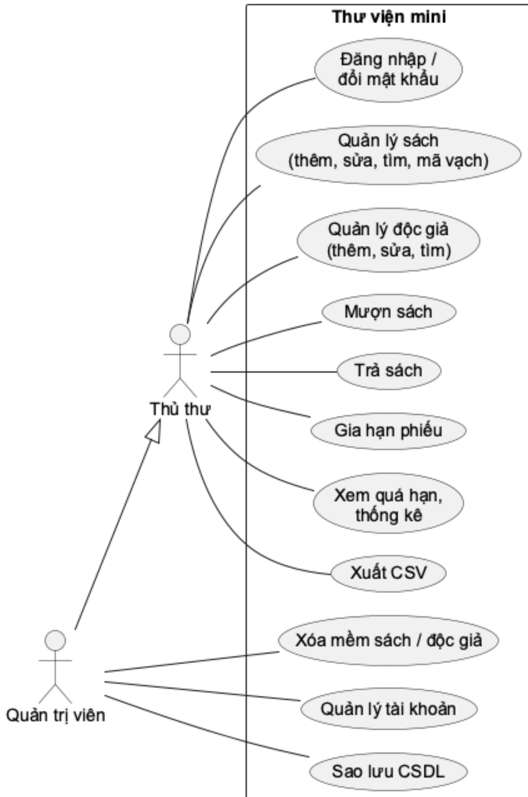
Hình 1. Tác nhân và chức năng hệ thống
