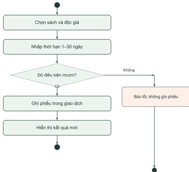
Hình 8. Luồng điều khiển mượn sách
