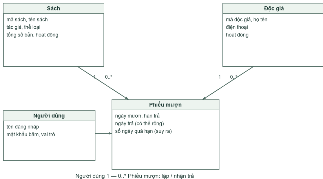
Hình 2. Lớp phân tích và quan hệ một–nhiều
