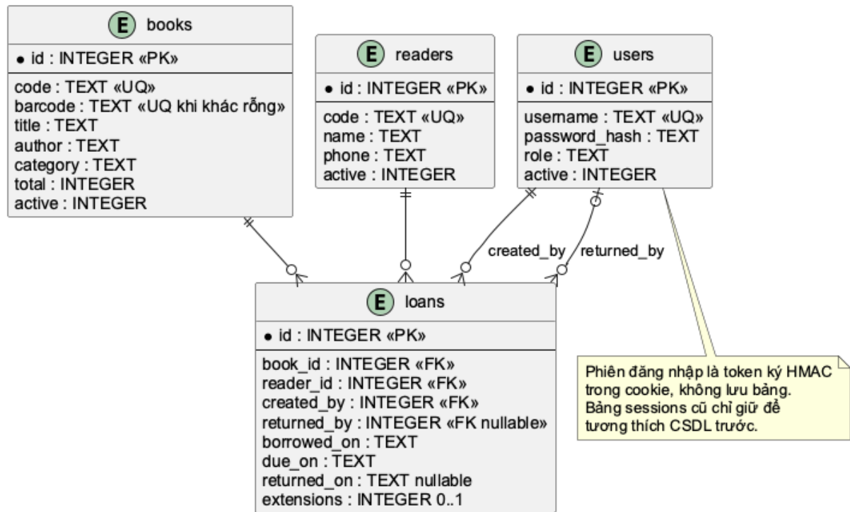
Hình 7. Lược đồ quan hệ SQLite
