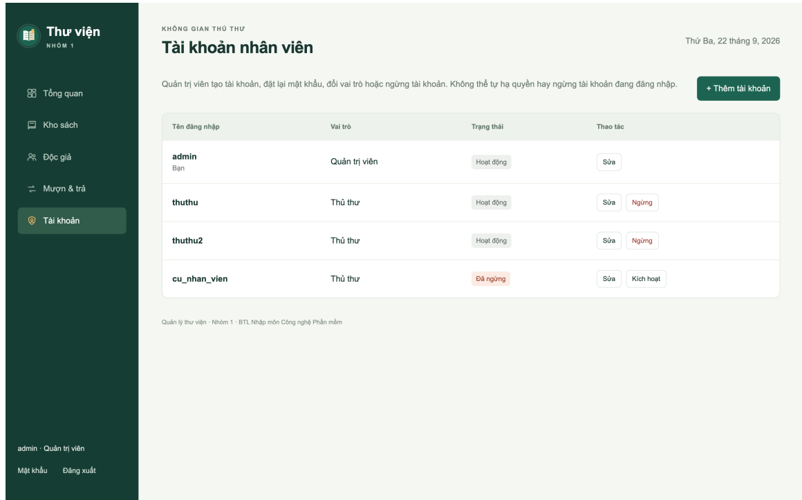
Hình 28. Màn hình Tài khoản
