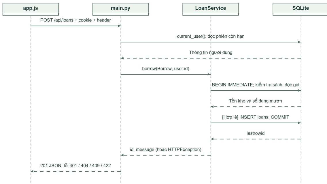
Hình 15. Ảnh xạ UC04 tới route, service và SQLite
