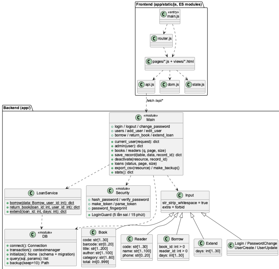
Hình 6. Các gói chức năng, DTO và lớp xử lý nghiệp vụ
