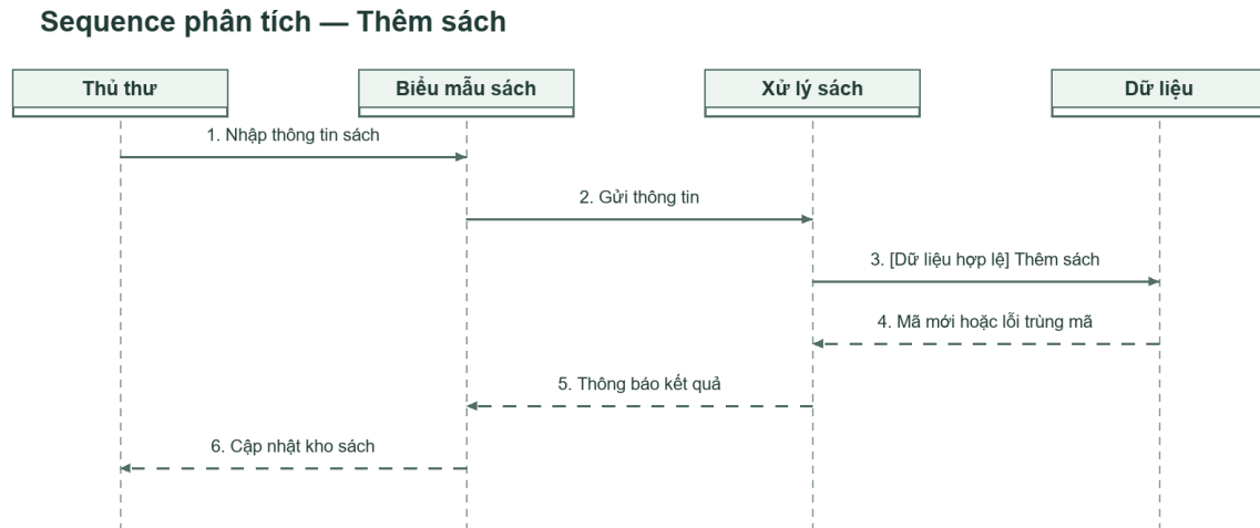
Hình 18. Tương tác thêm sách trong UC02
