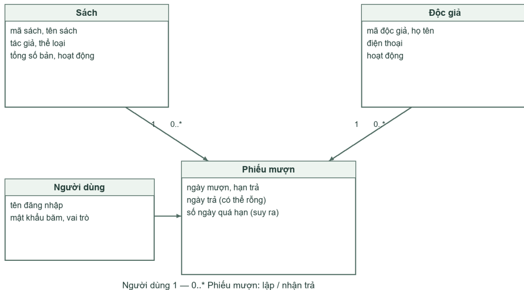
Hình 5. Lớp phân tích và quan hệ một-nhiều
