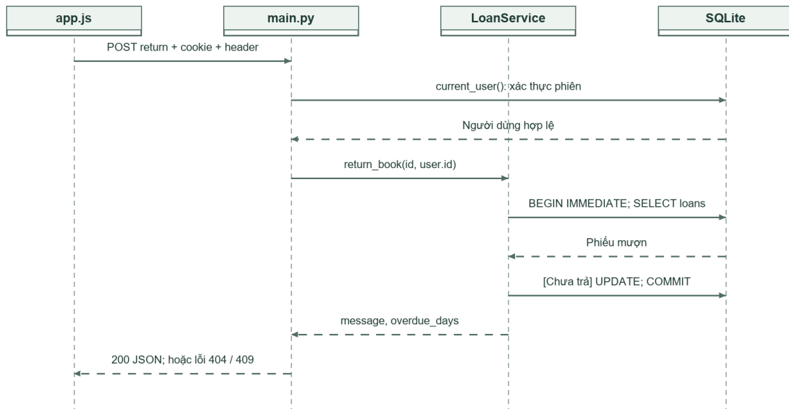
Hình 17. Ánh xạ UC05 tới route, service và SQLite
