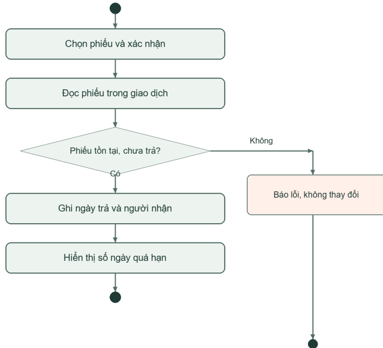
Hình 3. Luồng điều khiển trả sách
