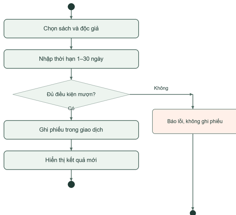
Hình 2. Luồng điều khiển mượn sách
