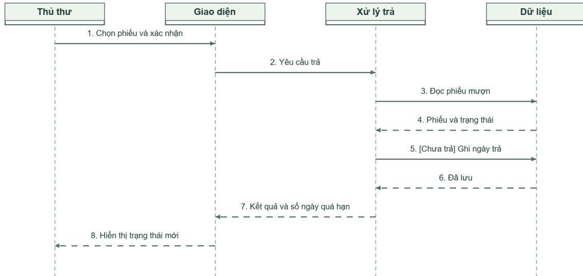
Hình 16. Tương tác nghiệp vụ UC05 Trả sách
