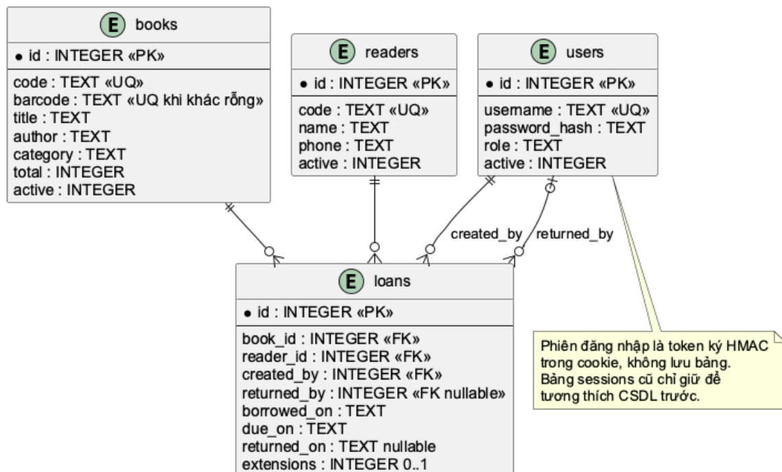
Hình 4. Lược đồ quan hệ SQLite
