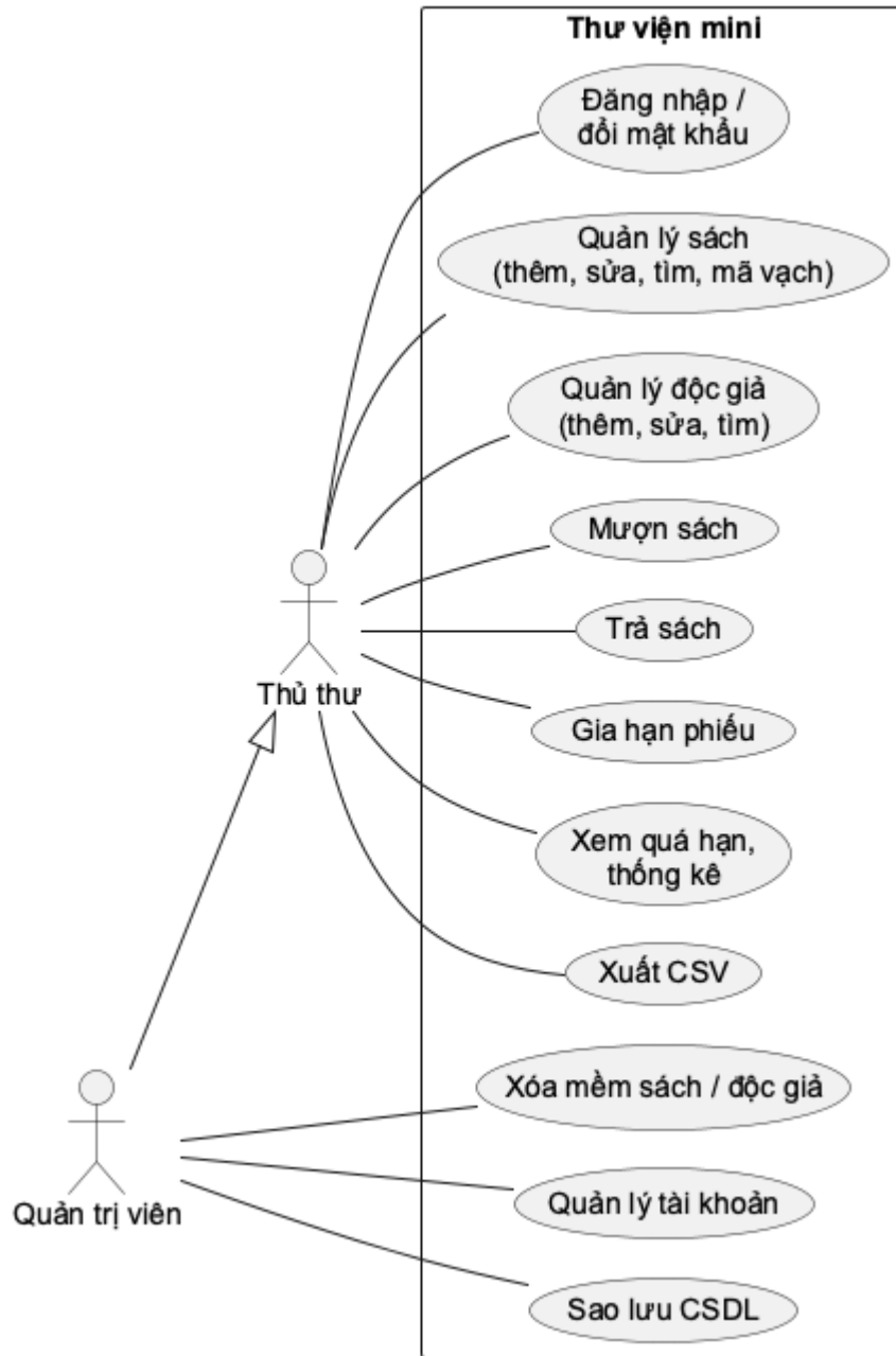
Hình 1. Tác nhân và chức năng hệ thống
