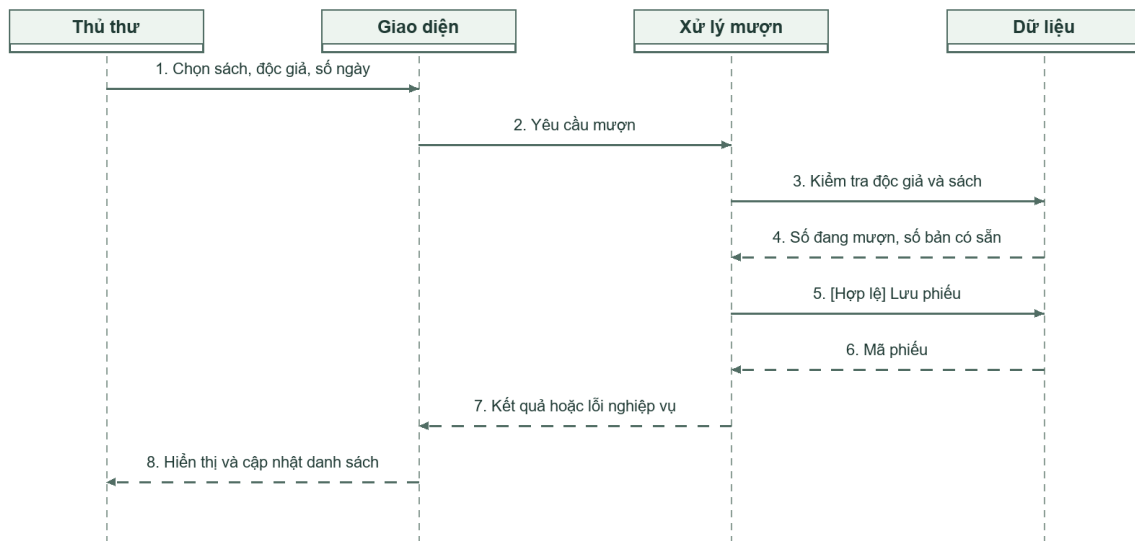
Hình 14. Tương tác nghiệp vụ UC04 Mượn sách
