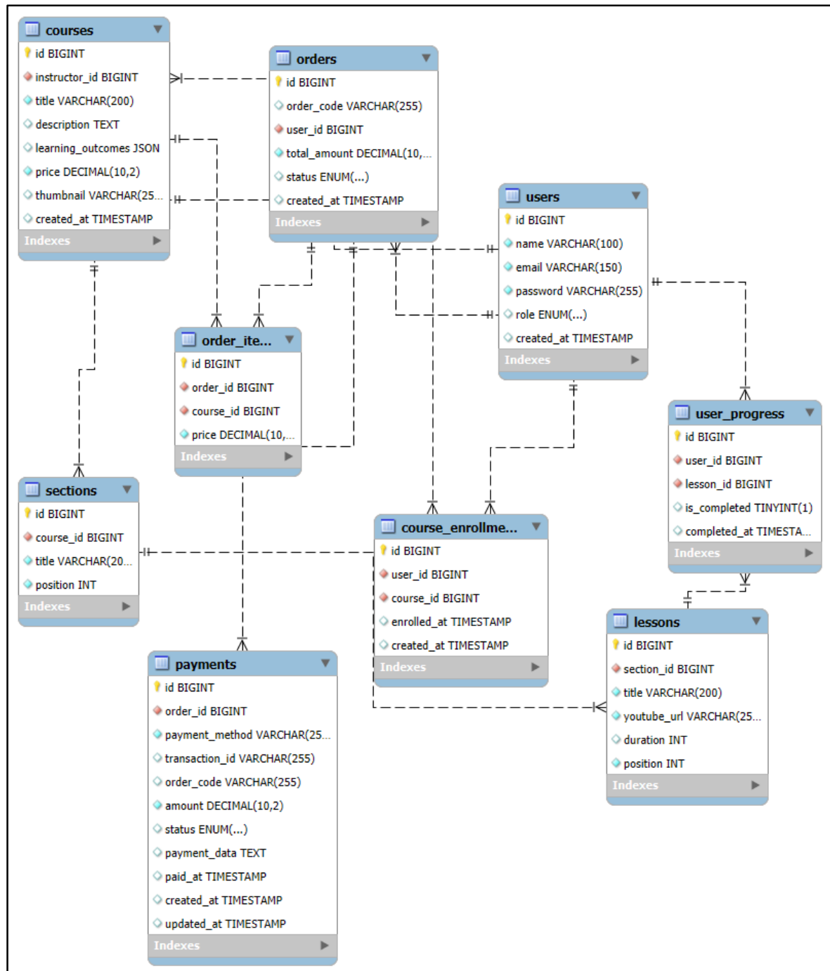
Hình 2. 5 Lược đồ cơ sở dữ liệu
