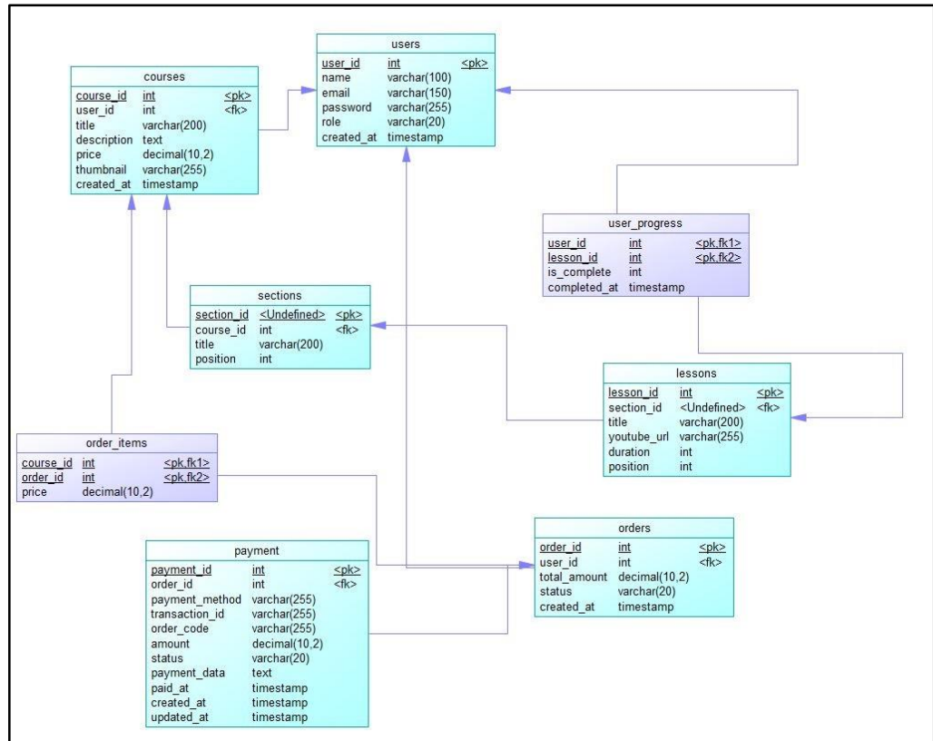
Hình 2. 3 Mô hình dữ liệu mức vật lý
