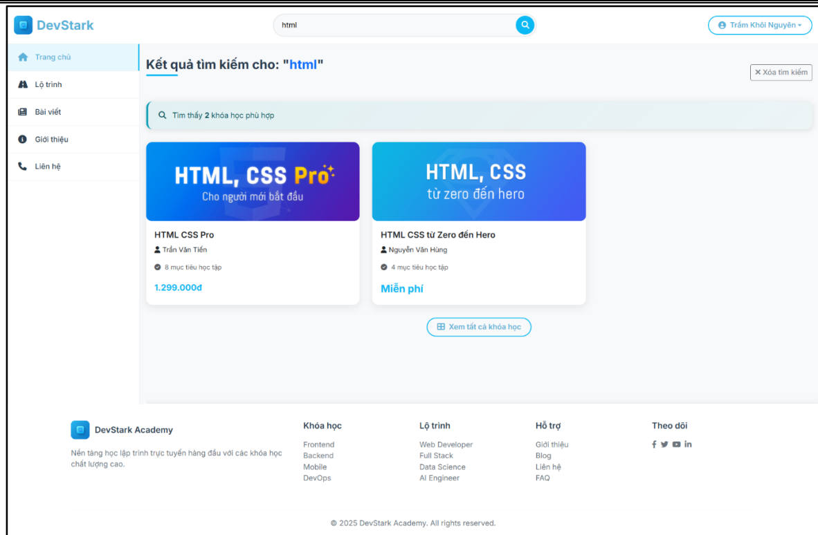
Hình 3. 7 Giao diện trang tìm kiếm khóa học
