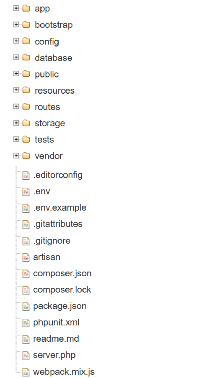
Hình 1. 1 Cấu trúc thư mục của Laravel Framework
