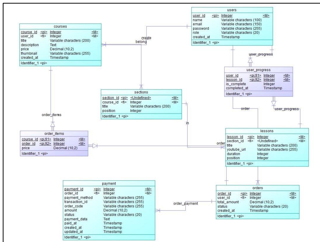
Hình 2. 2 Mô hình dữ liệu mức logic
