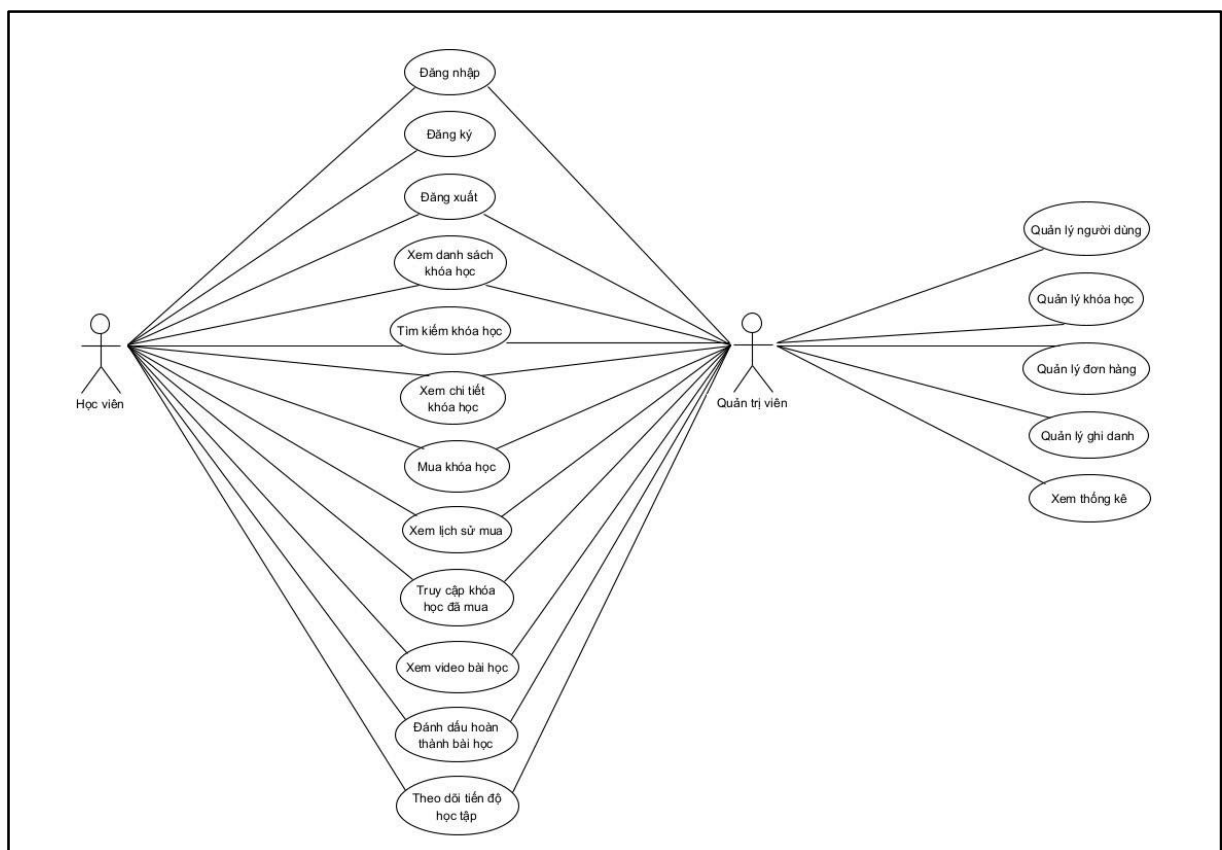
Hình 2. 4 Mô hình Use Case
