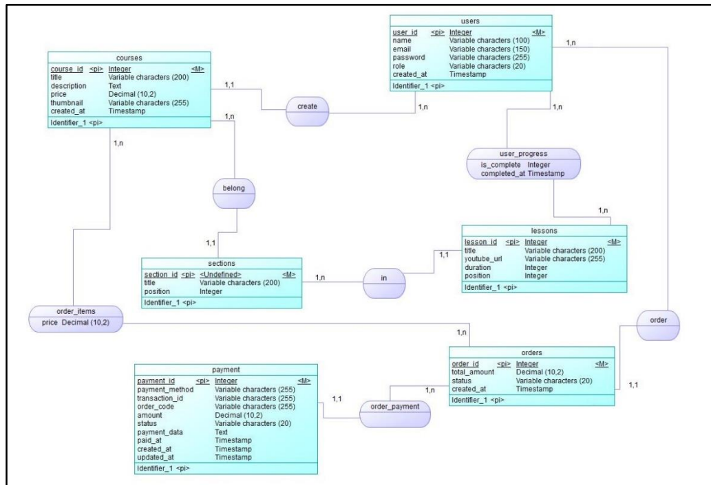
Hình 2. 1 Mô hình dữ liệu mức quan niệm
