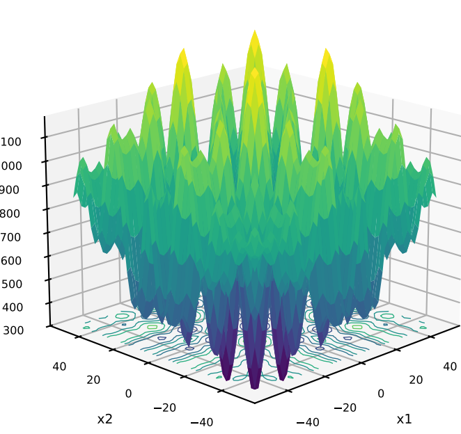
17: SchafferF7Cond1000
