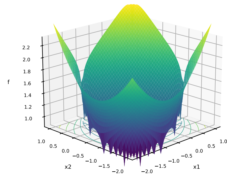
31: Step
