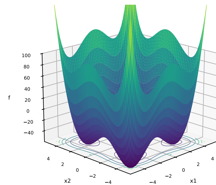
34: StyblinskiTang
