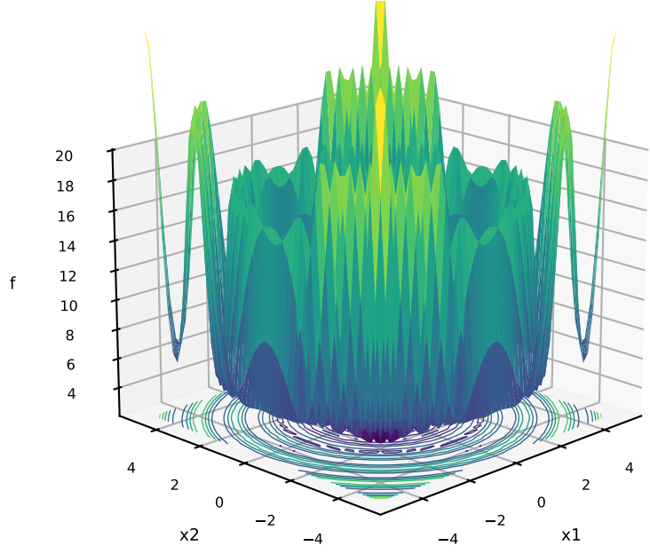
20: Katsuura
