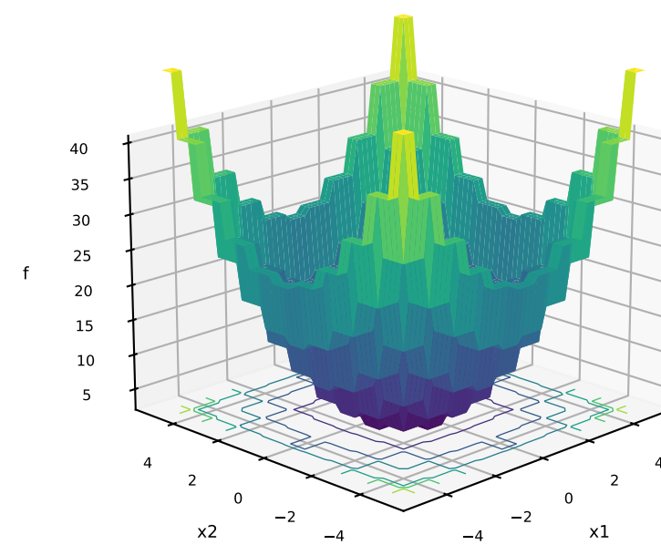
31: Step
