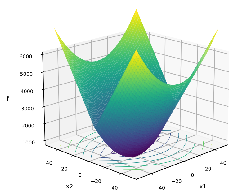
18: GriewankRosenbrock
