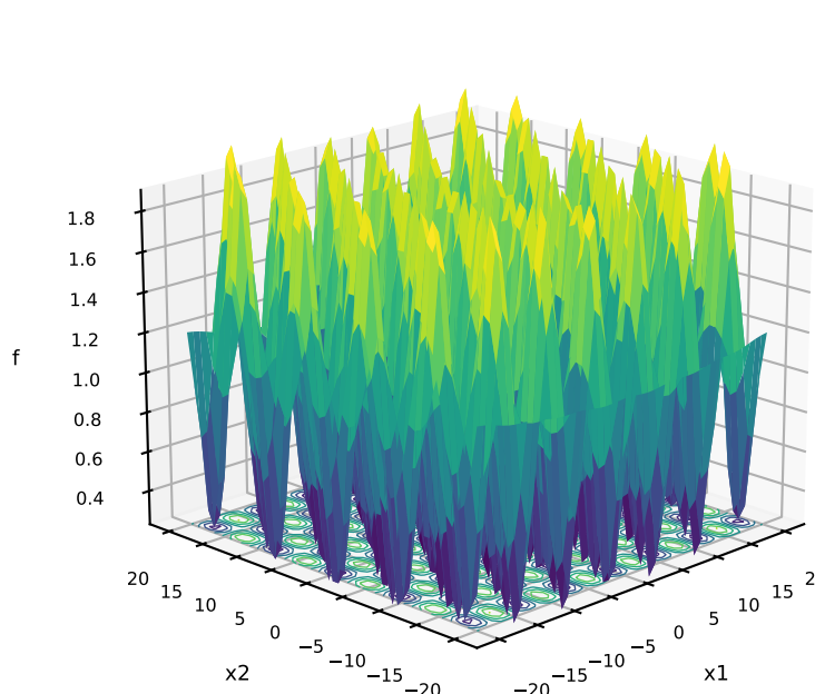
16: SchafferF7
