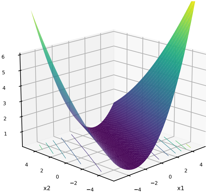
13: Schwefel
