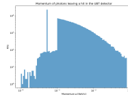
\gamma : \mathcal{O}(10) MeV/c
