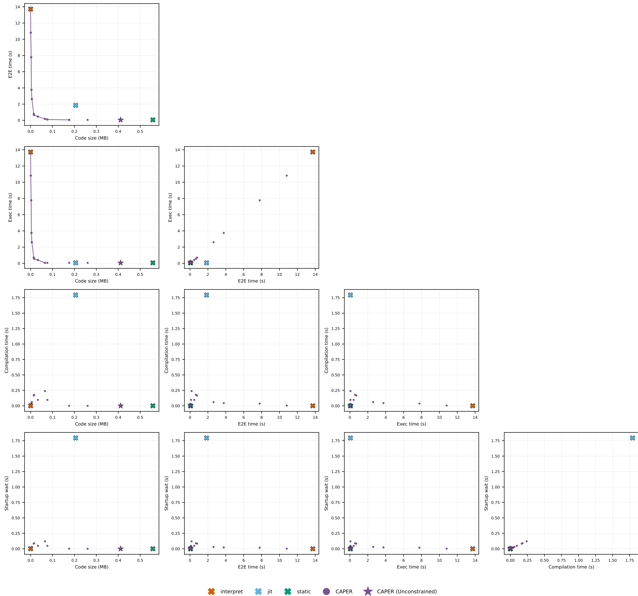
bzip2 · bzip2: pairwise metric trade-offs
