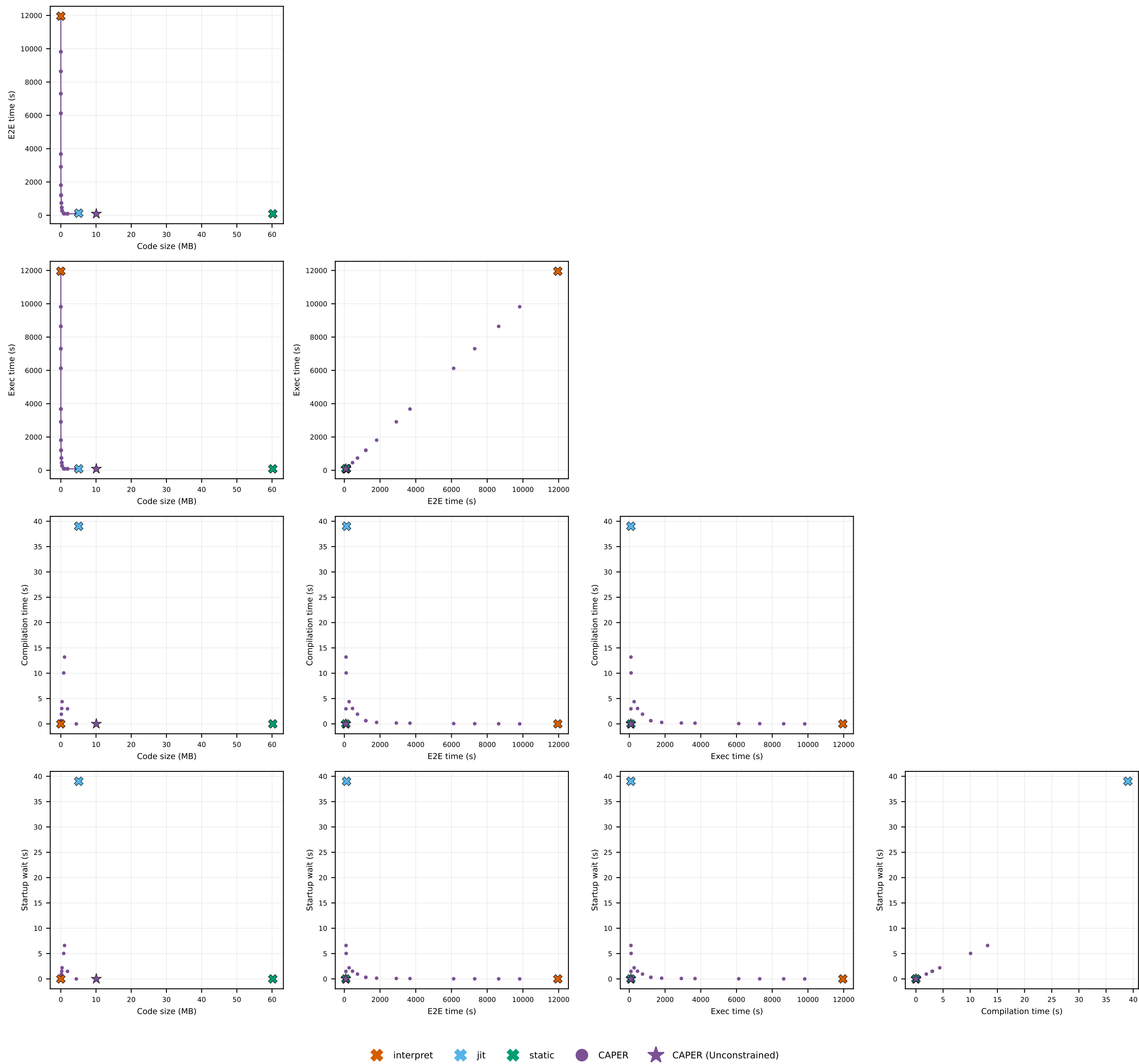
FFmpeg · mp4-flip-vertical: pairwise metric trade-offs
