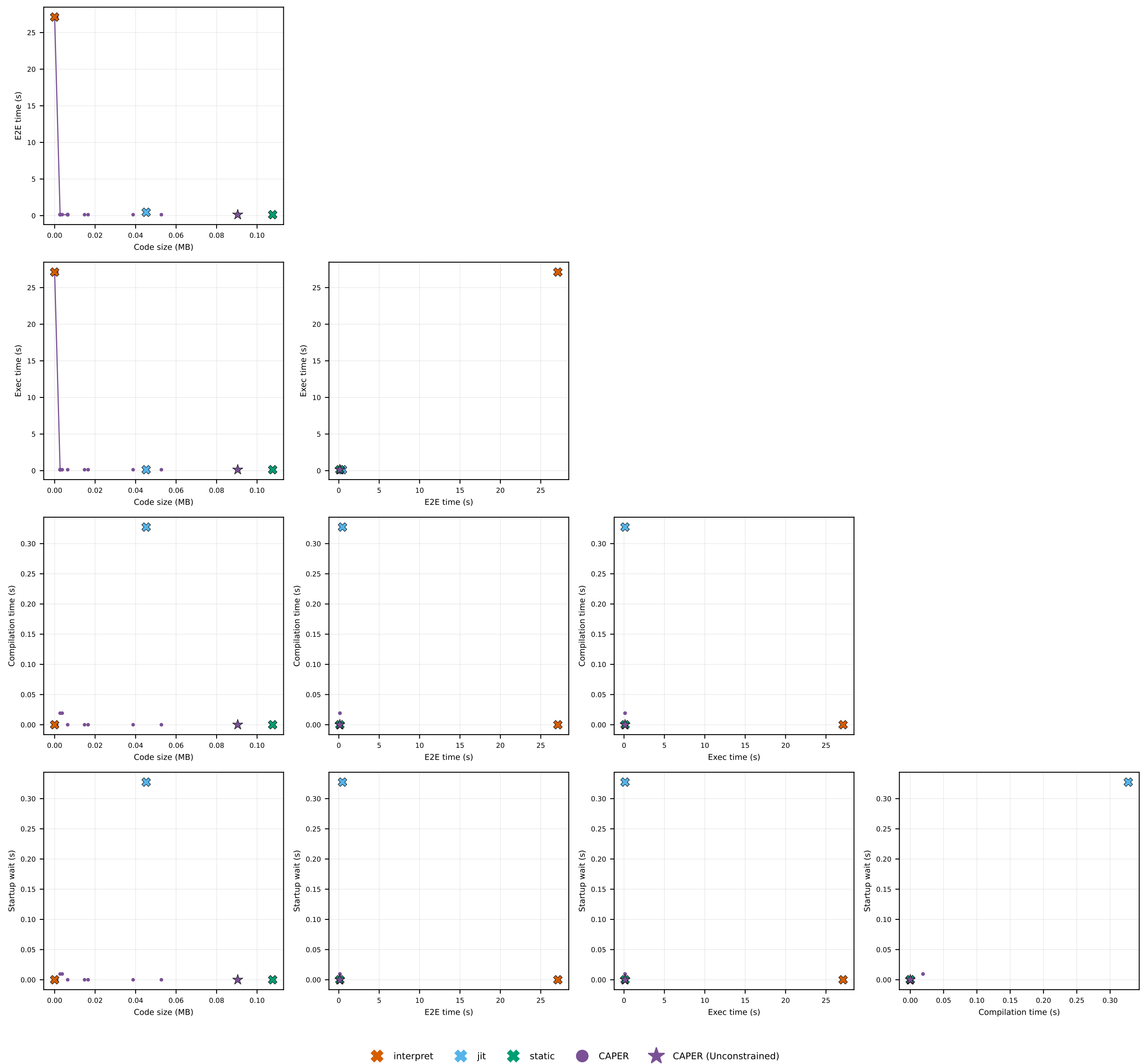
float-mm · float-mm: pairwise metric trade-offs
