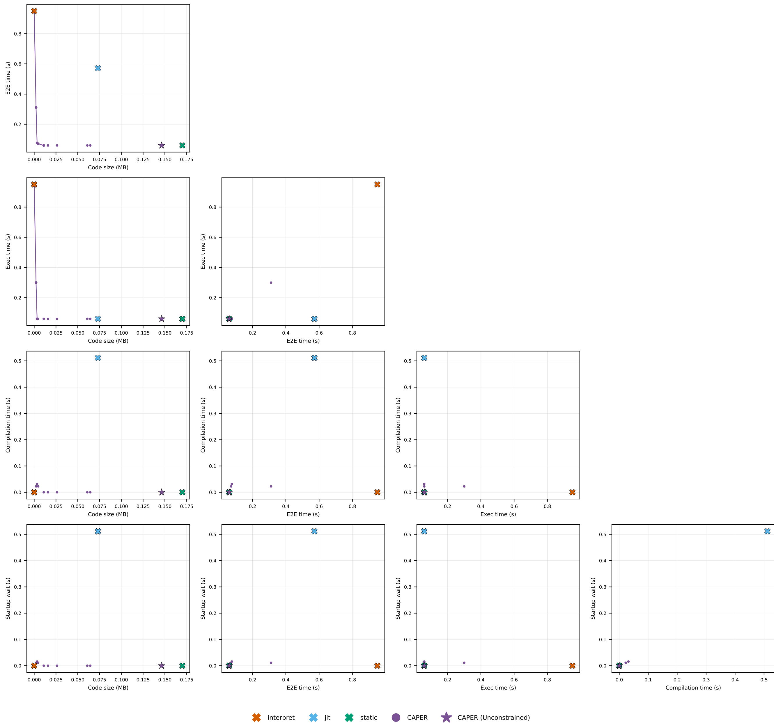
gemm · gemm: pairwise metric trade-offs
