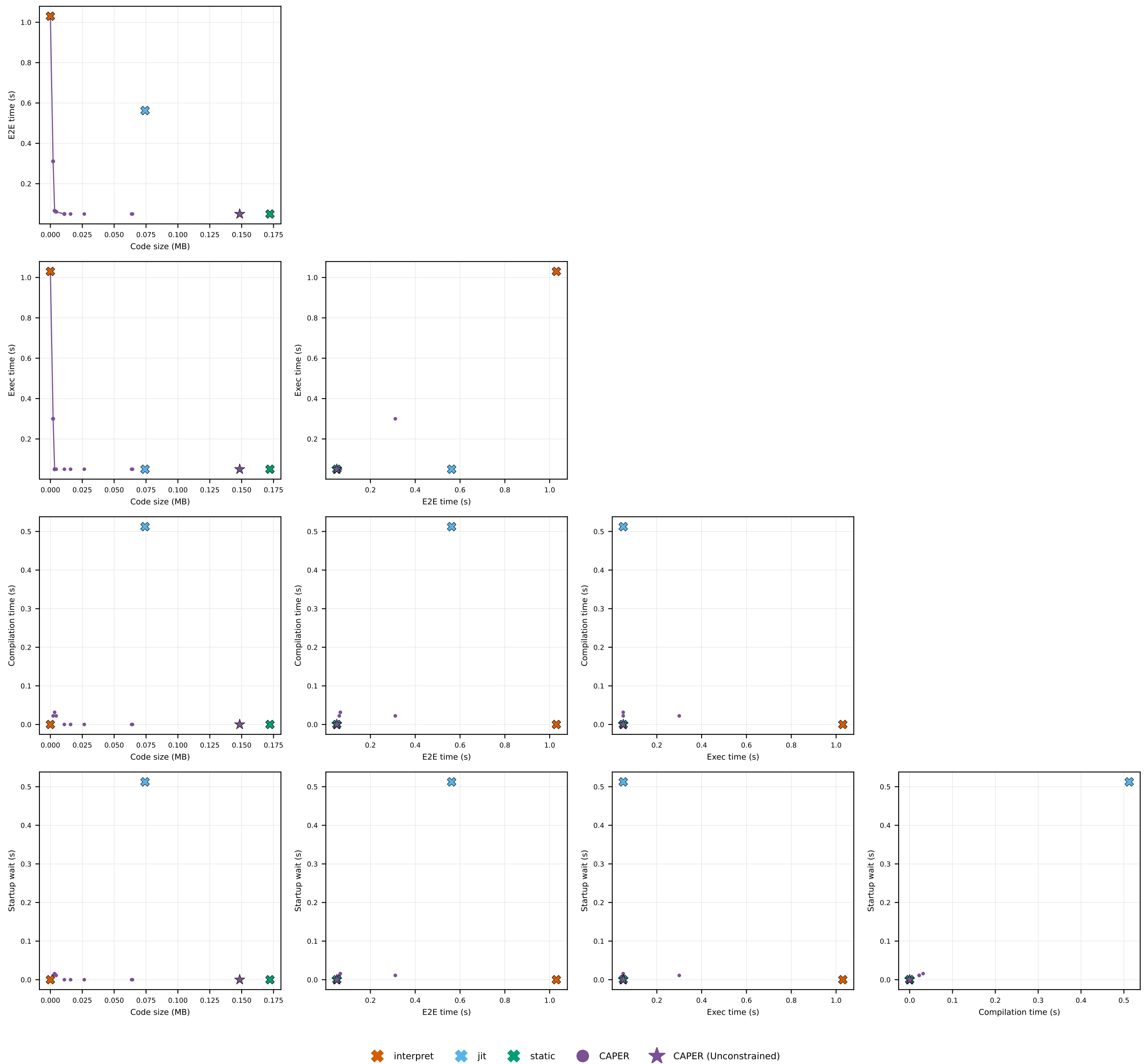
gemver · gemver: pairwise metric trade-offs
