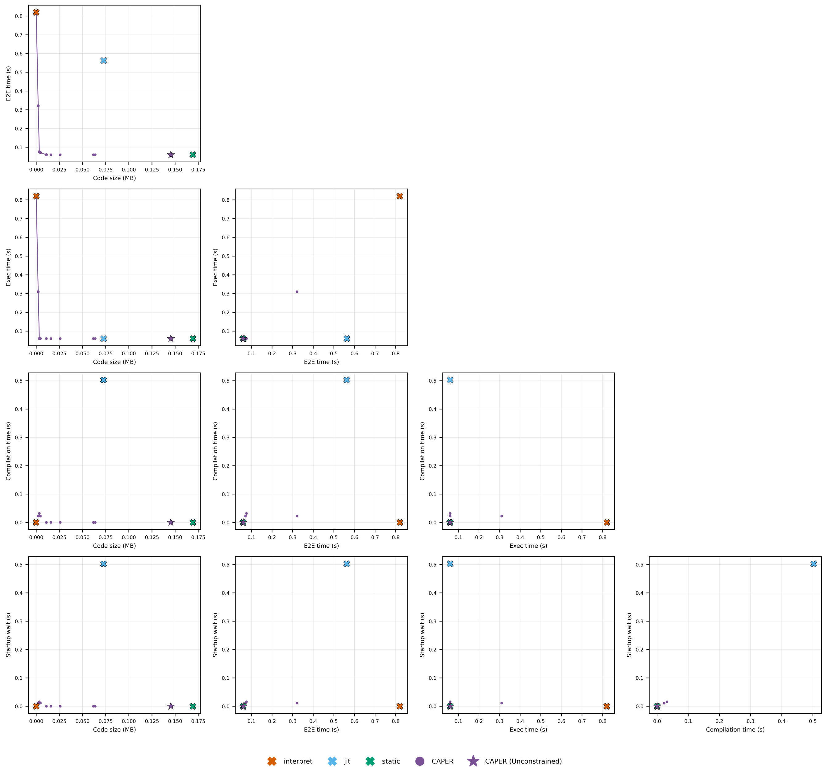
jacobi-2d · jacobi-2d: pairwise metric trade-offs
