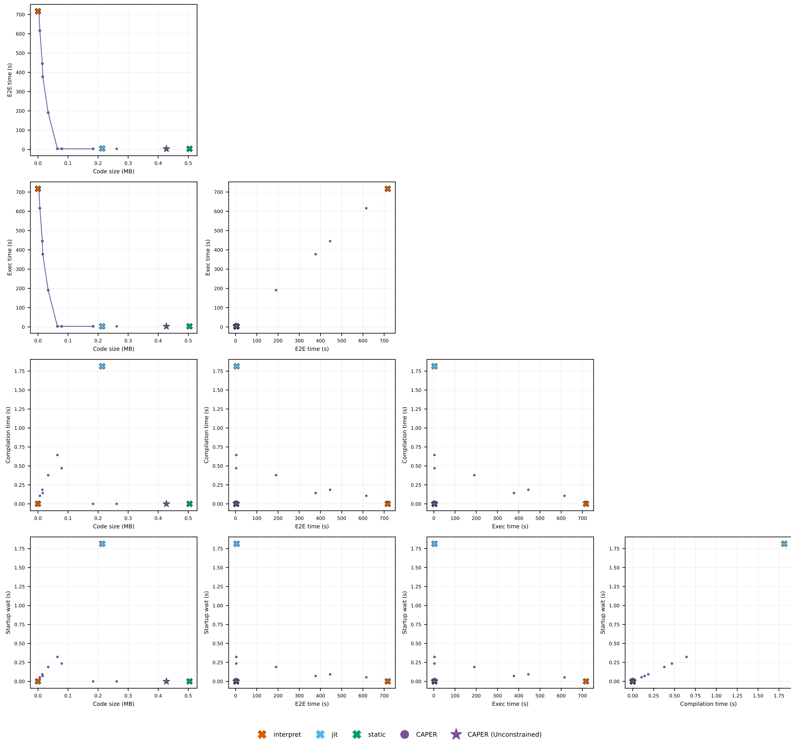
lu · lu: pairwise metric trade-offs
