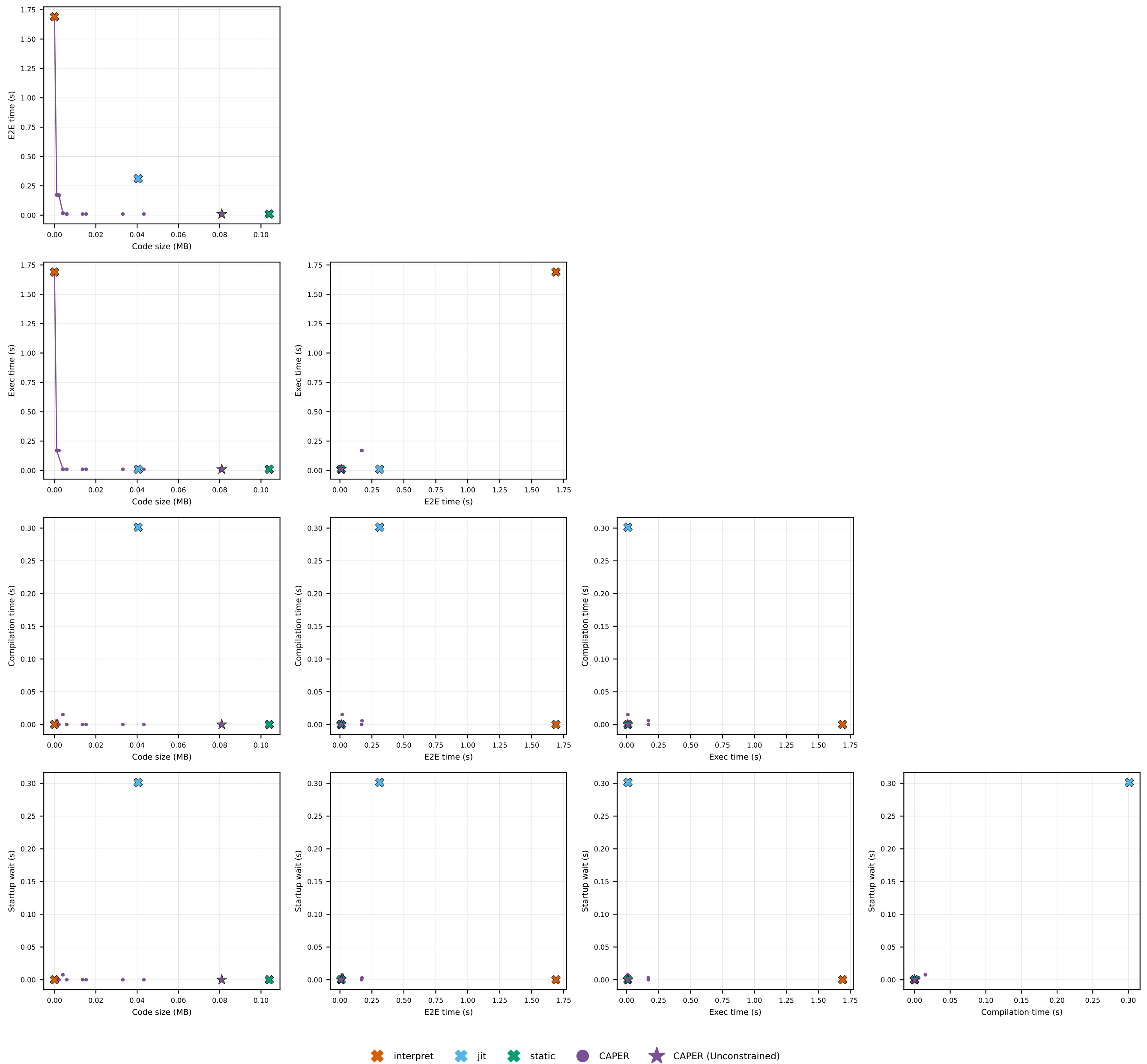
quicksort · quicksort: pairwise metric trade-offs
