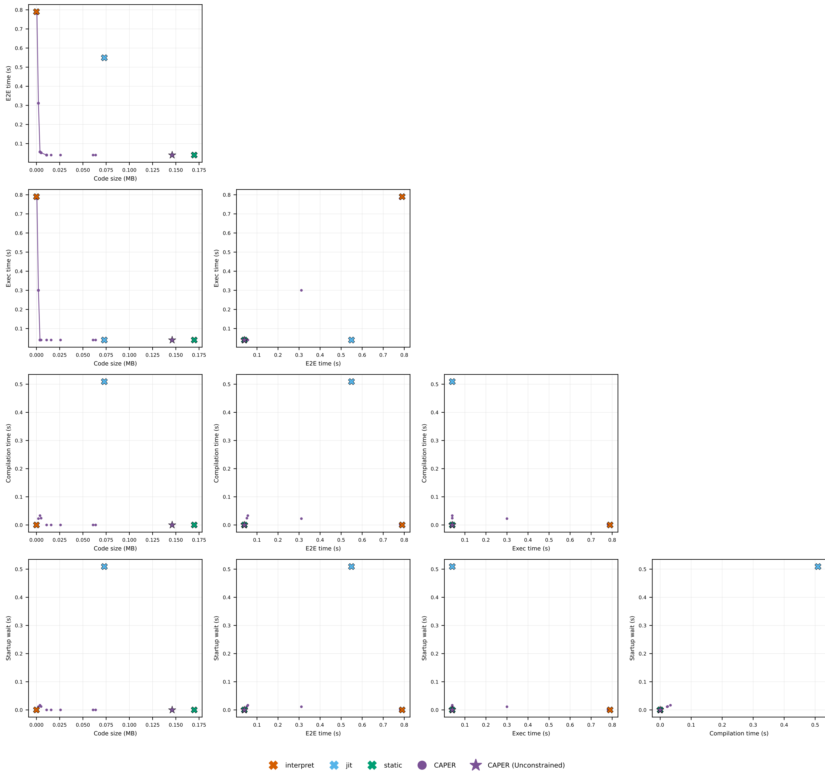
syrk · syrk: pairwise metric trade-offs
