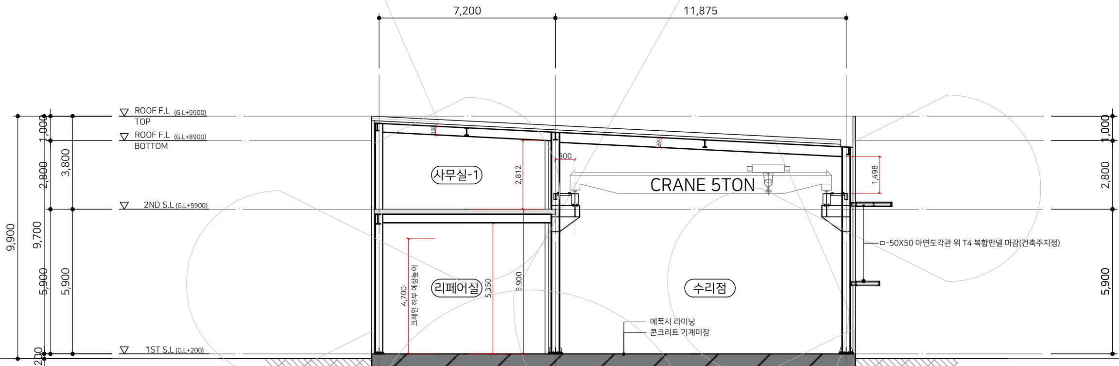
1 A301 종단면도-1 SCALE _ A1 1 / 75 , A3 1 / 150
