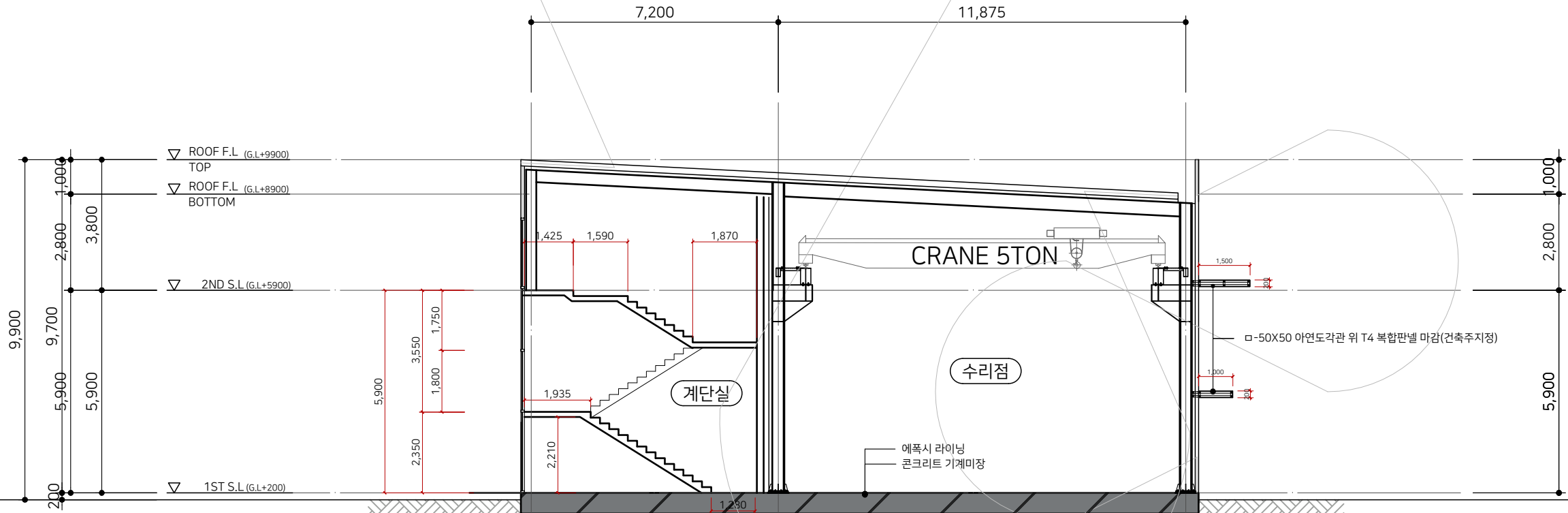
1 A301 종단면도-2 SCALE _ A1 1 / 75 , A3 1 / 150
