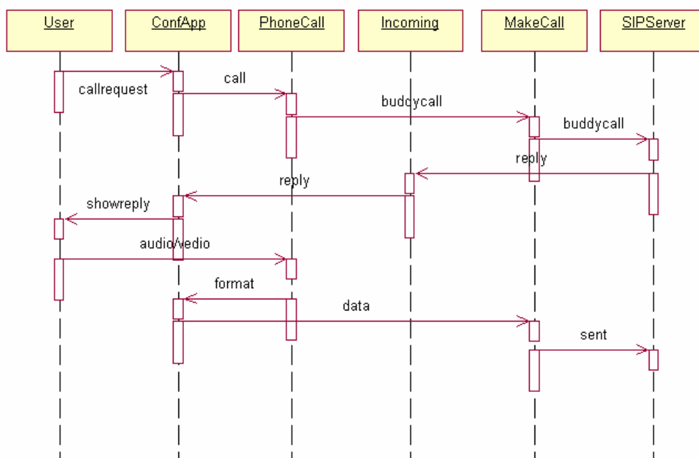
รูปที่ 4.2.8 แสดงลำดับขั้นตอนการทำงานของ การติดต่อแบบ PhoneCall
