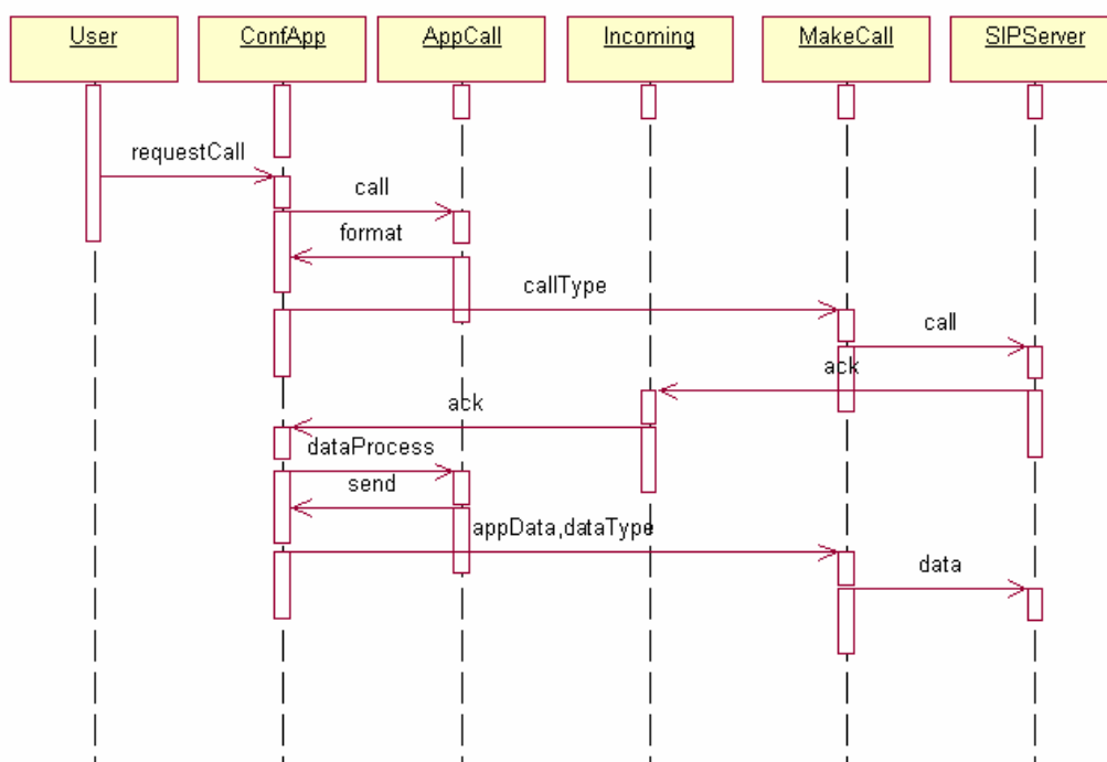
รูปที่ 4.2.7 แสดงลำดับขั้นตอนการทำงานของ การติดต่อแบบ AppCall
