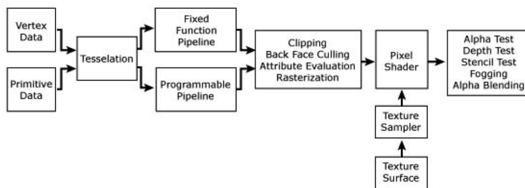
รูปที่ 3-6 รูปแสดง Pipeline การทำงานของ Direct3D
