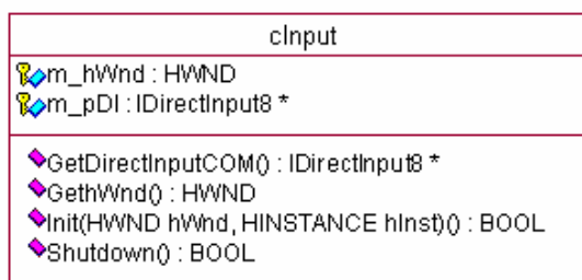
รูปที่ 7-1 คลาสไคอะแกรมของ cInput
