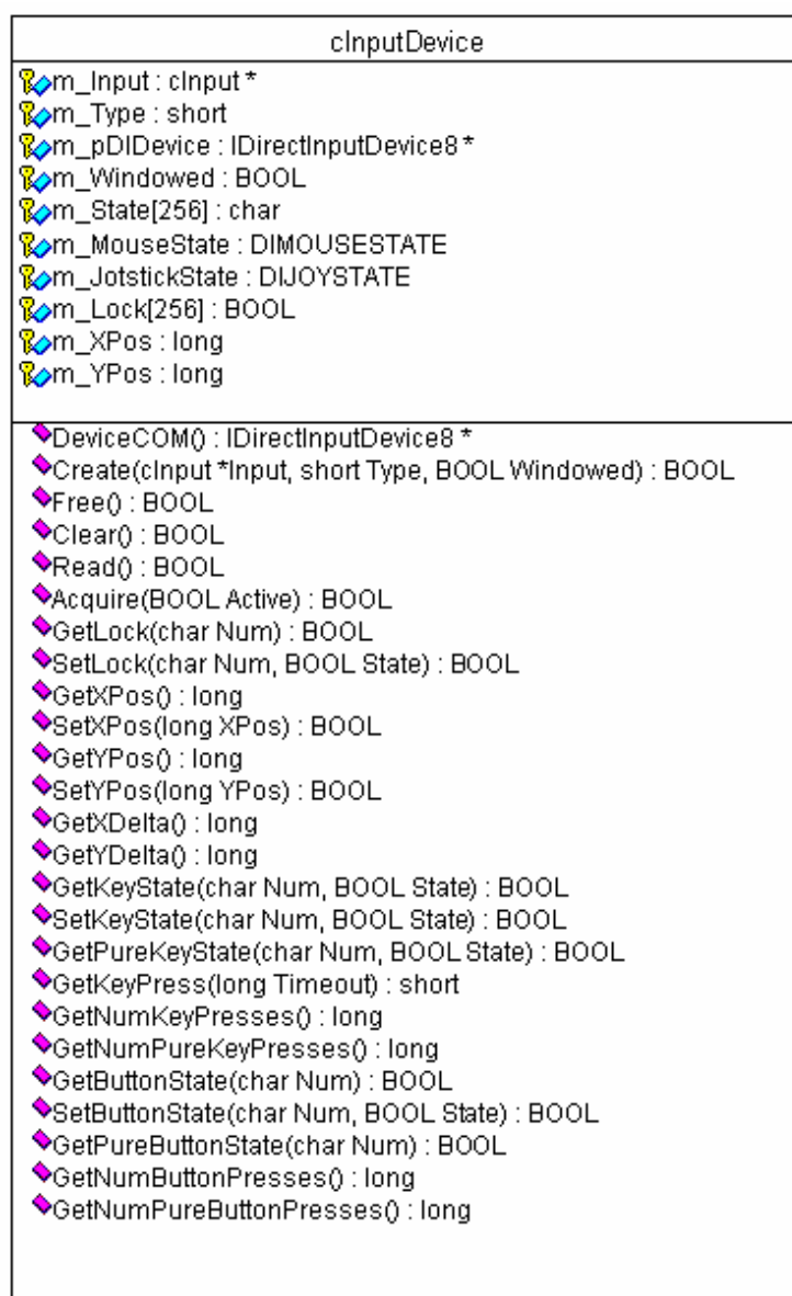
รูปที่ 7-2 คลาสไลอะแกรมของ cInputDevice
