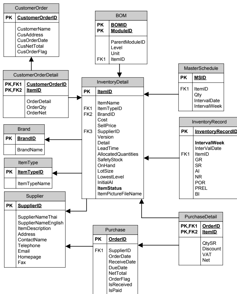
รูปที่ 1-1 แสดงการออกแบบฐานข้อมูลโดยใช้ ER Schema
