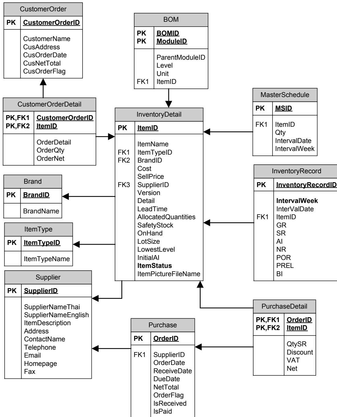
รูปที่ 5-5 แสดงการออกแบบฐานข้อมูลโดยใช้ ER Schema
