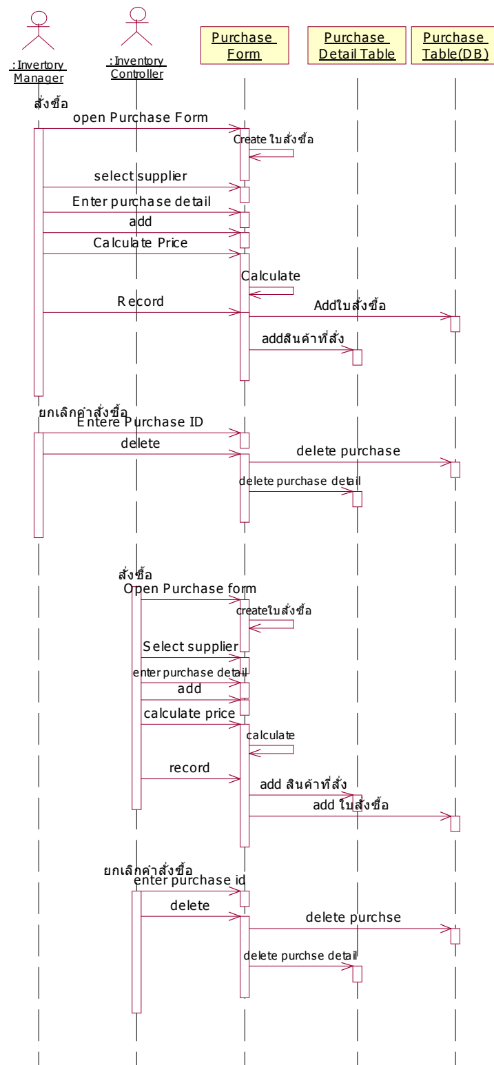
รูปที่ 5-10 แสดงการออกแบบ Sequence Diagram ของการสั่งวัสดุ
