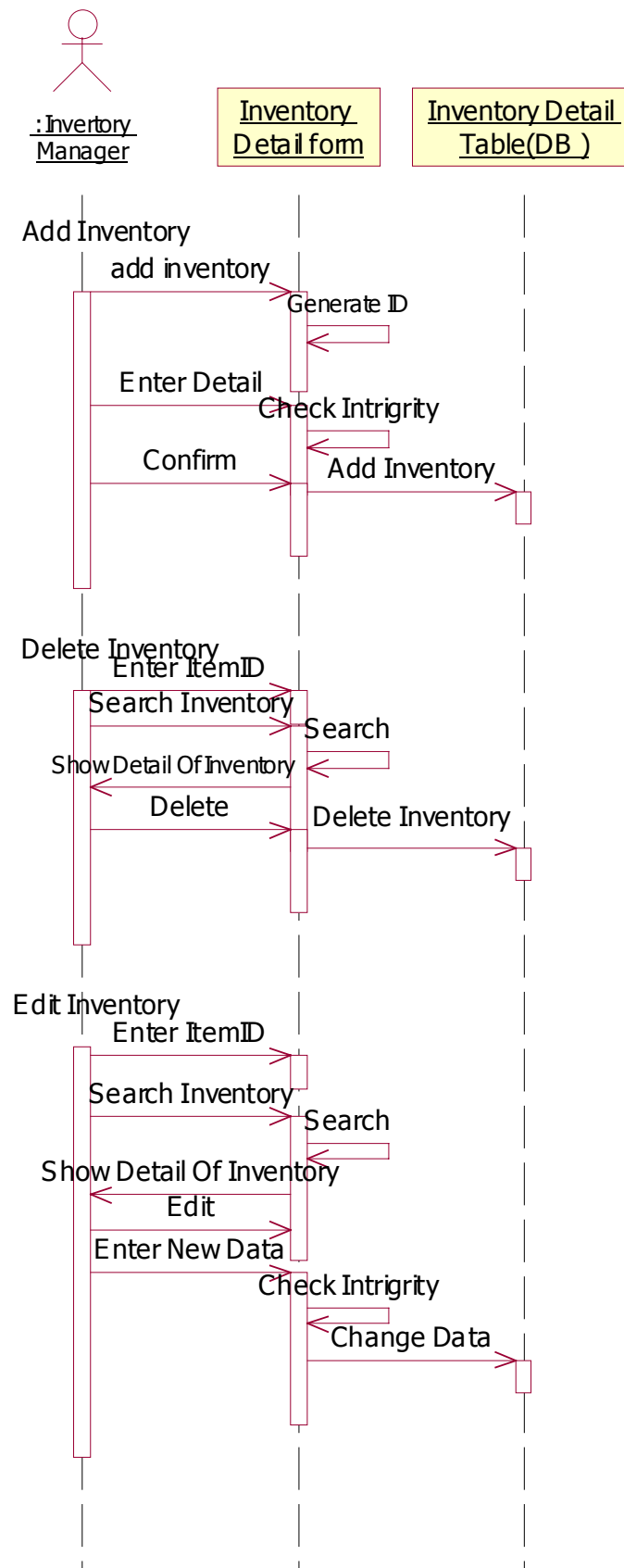
รูปที่ 5-13 แสดงการออกแบบ Sequence Diagram ของการจัดการรายละเอียดของคลัง
