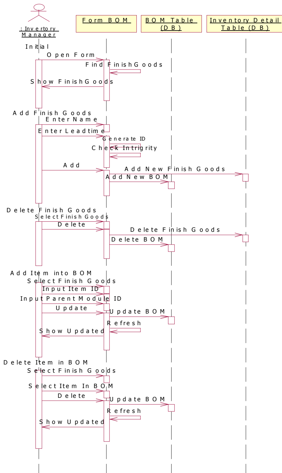
รูปที่ 5-7 แสดงการออกแบบ Sequence Diagram ของ Bill of Material
