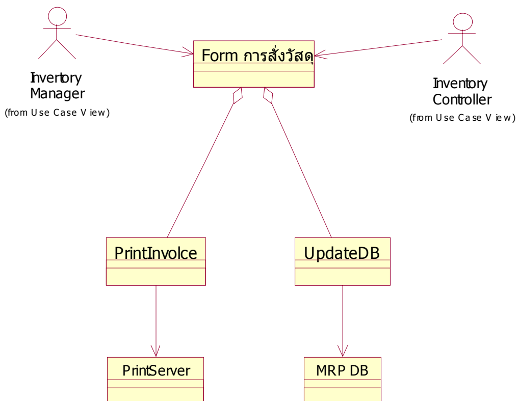
รูปที่ 5-20 แสดงการออกแบบ Class Diagram ของการสั่งวัสดุ
