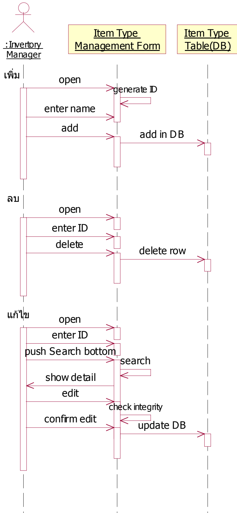
รูปที่ 5-16 แสดงการออกแบบ Sequence Diagram ของการจัดการชนิดของสินค้าและวัตถุดิบ
