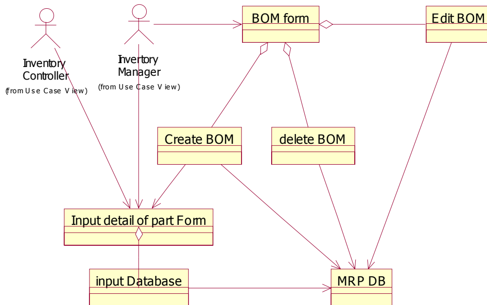
รูปที่ 5-17 แสดงการออกแบบ Class Diagram ของการเพิ่ม BOM
