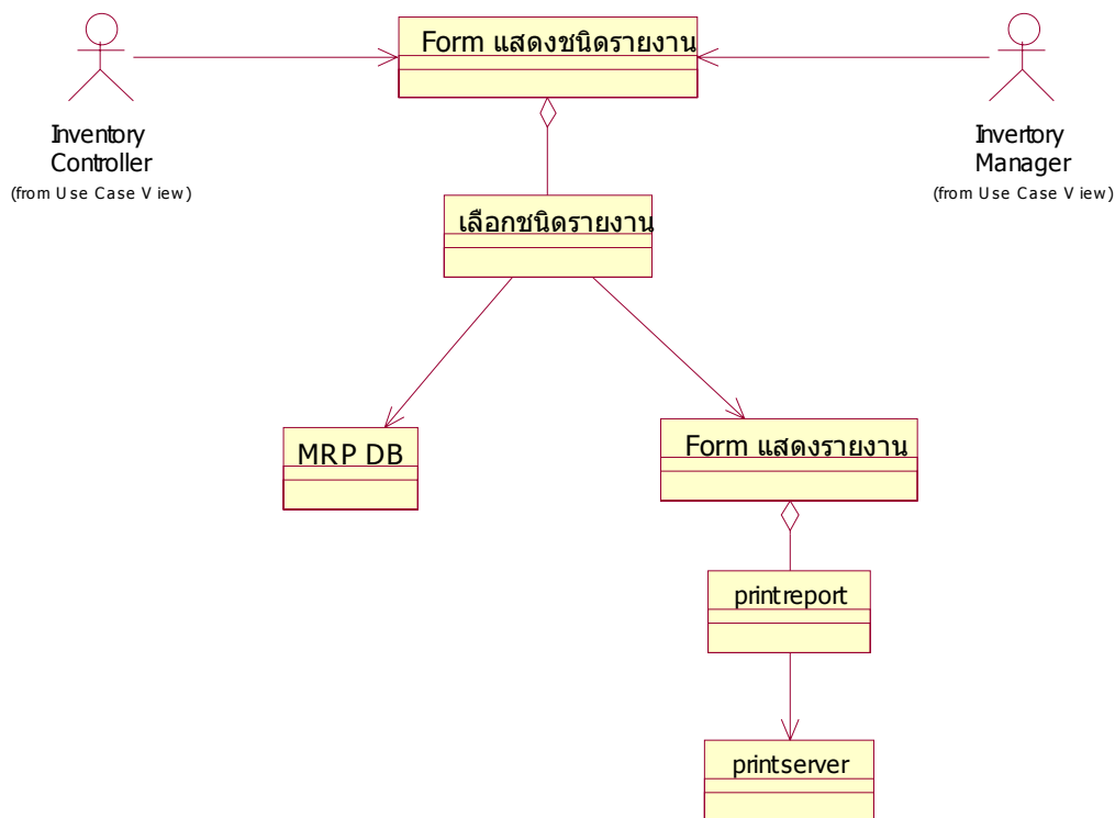
รูปที่ 5-21 แสดงการออกแบบ Class Diagram ของการออกรายงาน
