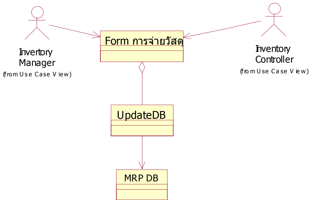
รูปที่ 5-19 แสดงการออกแบบ Class Diagram ของการเบิกจ่ายวัสดุ
