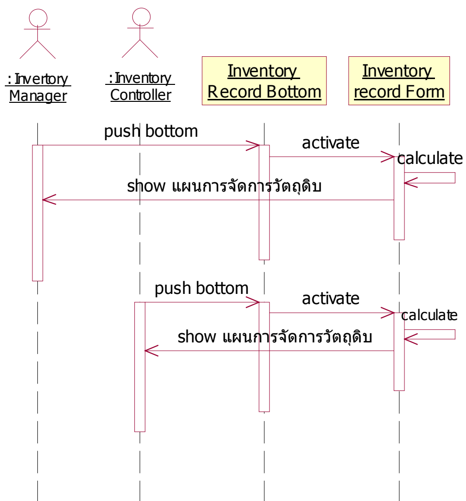
รูปที่ 5-9 แสดงการออกแบบ Sequence Diagram ของแผนการจัดการวัตถุดิบ
