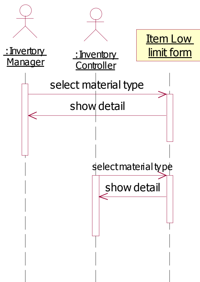
รูปที่ 5-15 แสดงการออกแบบ Sequence Diagram ของการตรวจสอบสินค้าที่เหลือน้อย
