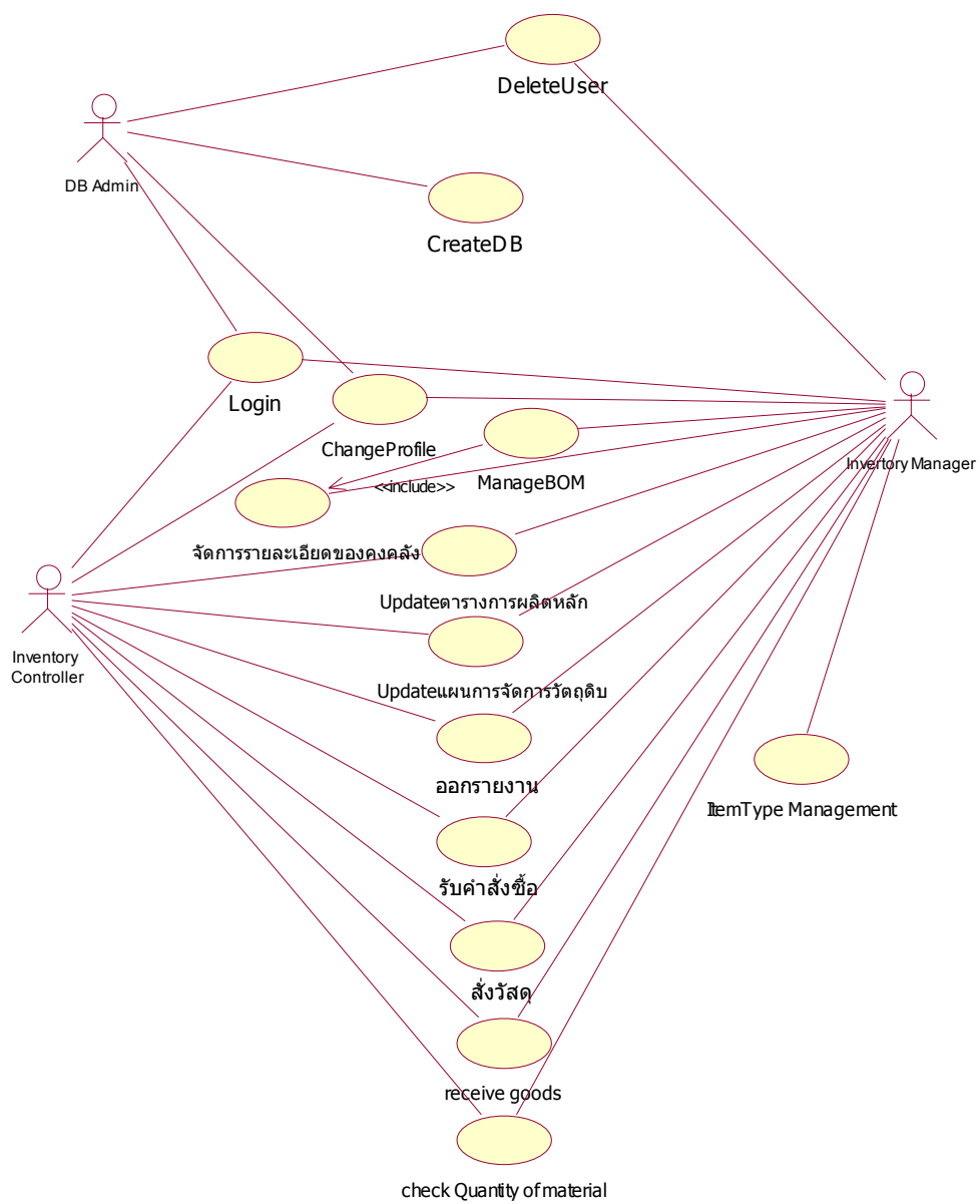
รูปที่ 5-6 แสดง USE CASE DIAGRAM ของระบบโดยรวม
