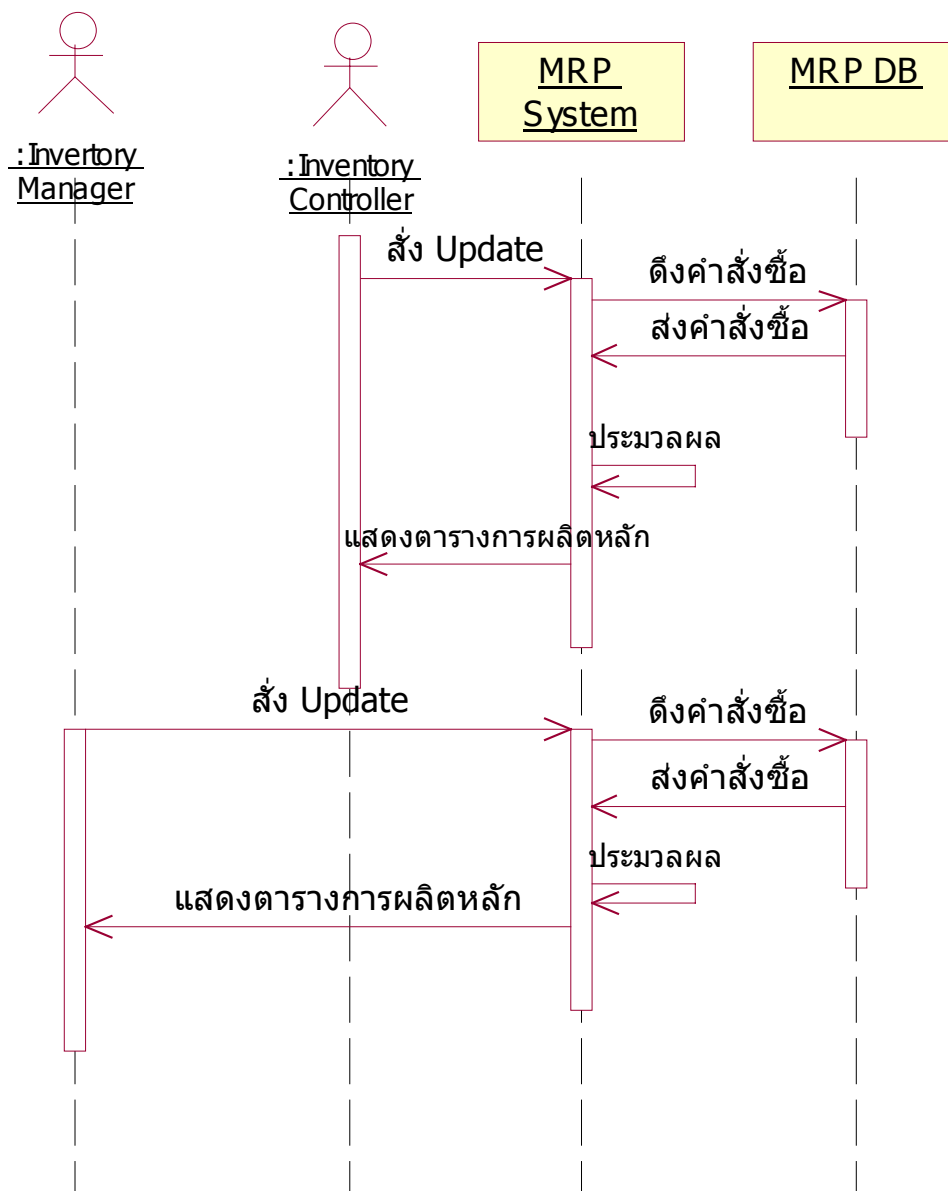
รูปที่ 5-8 แสดงการออกแบบ Sequence Diagram ของตารางการผลิตหลัก
