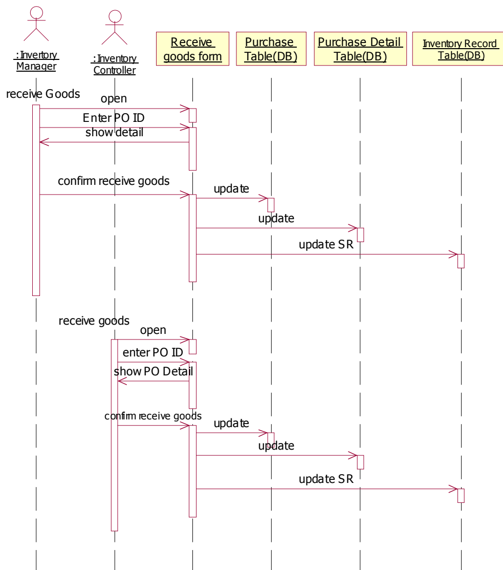
รูปที่ 5-14 แสดงการออกแบบ Sequence Diagram ของการรับสินค้า
