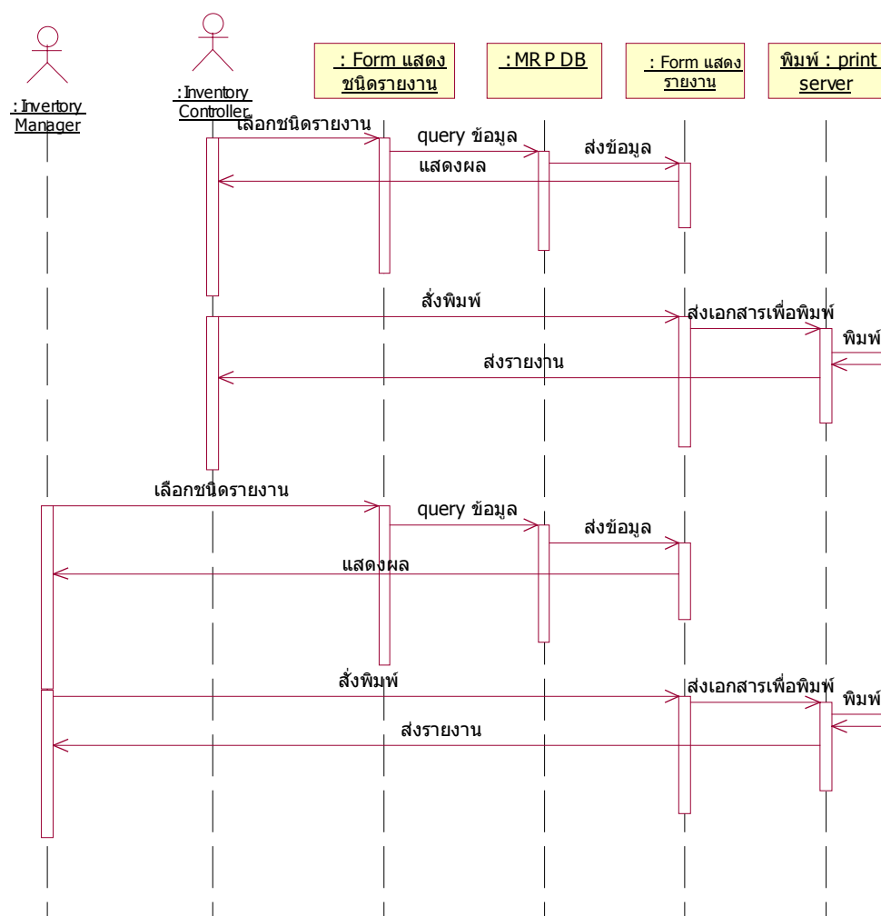
รูปที่ 5-11 แสดงการออกแบบ Sequence Diagram ของการออกรายงาน
