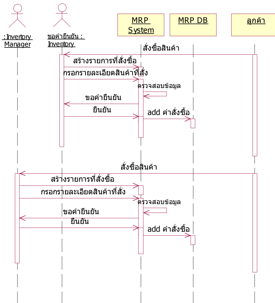
รูปที่ 5-12 แสดงการออกแบบ Sequence Diagram ของการรับคำสั่งซื้อ
