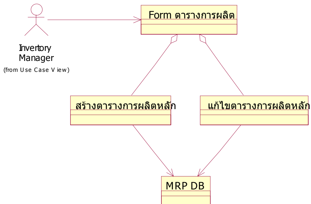
รูปที่ 5-18 แสดงการออกแบบ Class Diagram ของการสร้างตารางการผลิตหลัก
