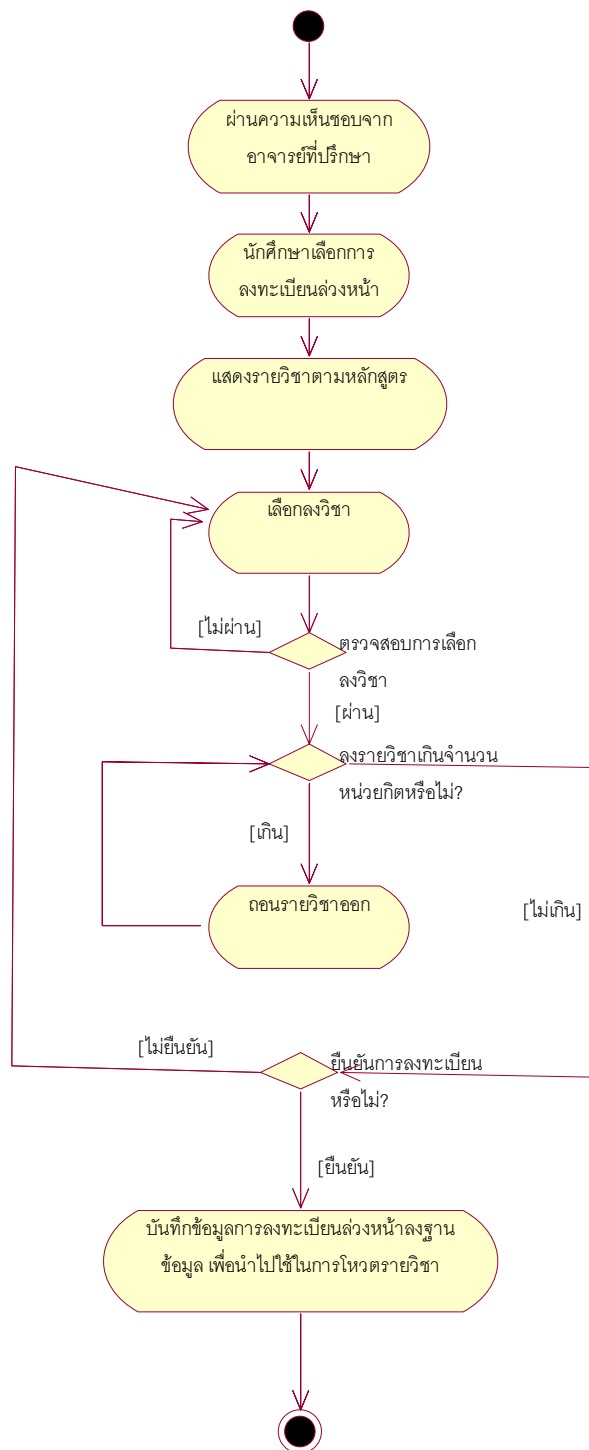
Activity Diagram ของ การลงทะเบียนล่วงหน้า
