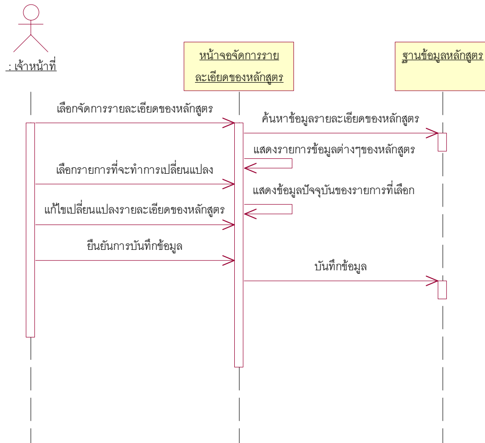
Sequence Diagram ของ การ จัดการรายละเอียดของหลักสูตร
