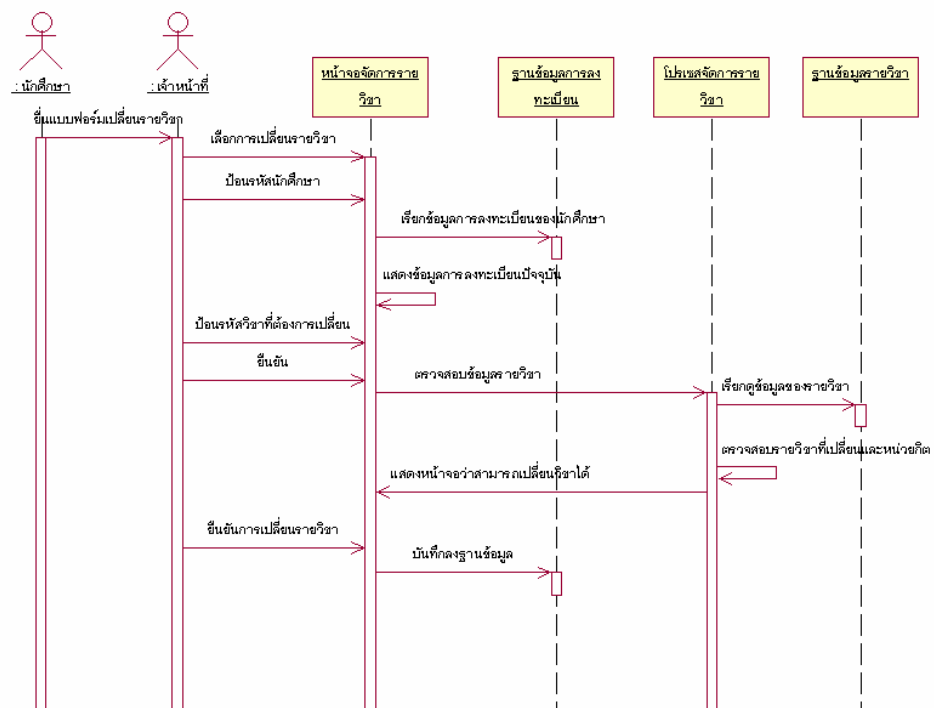
Sequence Diagram ของ การ เปลี่ยนรายวิชา
