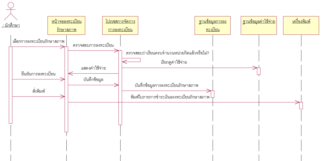
Sequence Diagram ของ การ ลงทะเบียนรักษาสุขภาพ
