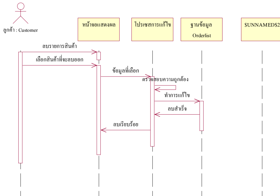
รูปที่ 8-10 แสดง Sequence diagram ของ การลบรายการสินค้า
