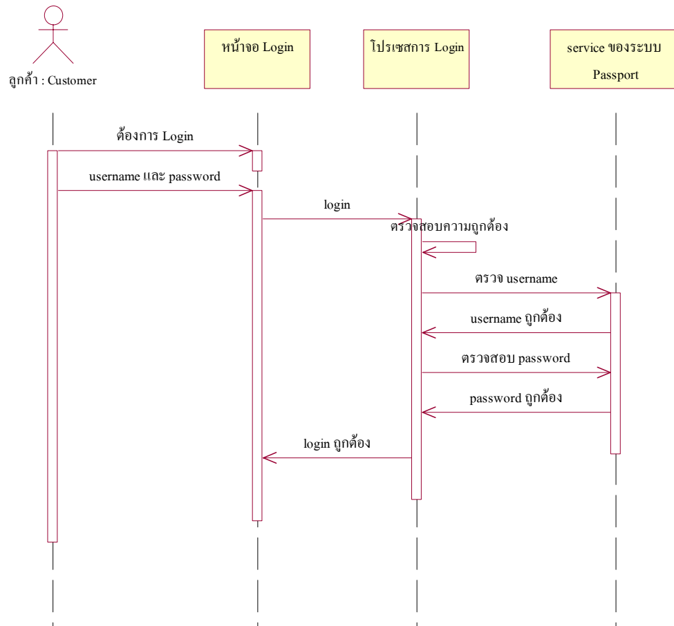
รูปที่ 8-3 แสดง Sequence diagram ของ Login
