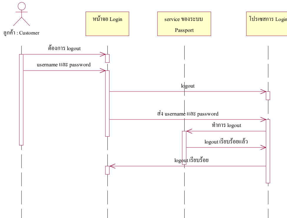
รูปที่ 8-4 แสดง Sequence diagram ของ Logout
