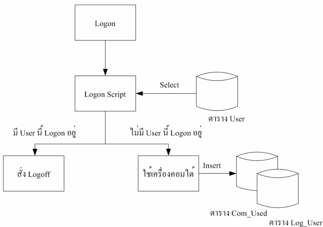
รูปที่ 1 แสดงขั้นตอนการทำงานของ Logon Scripts
