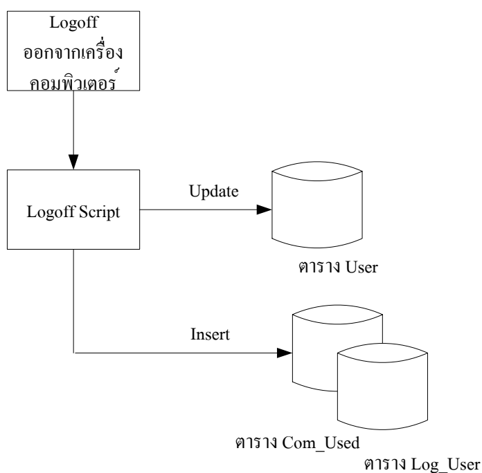
รูปที่ 2 แสดงขั้นตอนการทำงานของ Logoff Scripts
