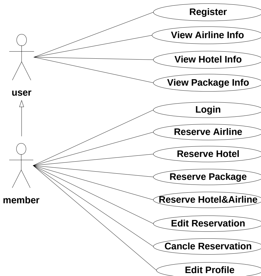
รูปที่ 6.3 Use Case Diagram ของระบบ
