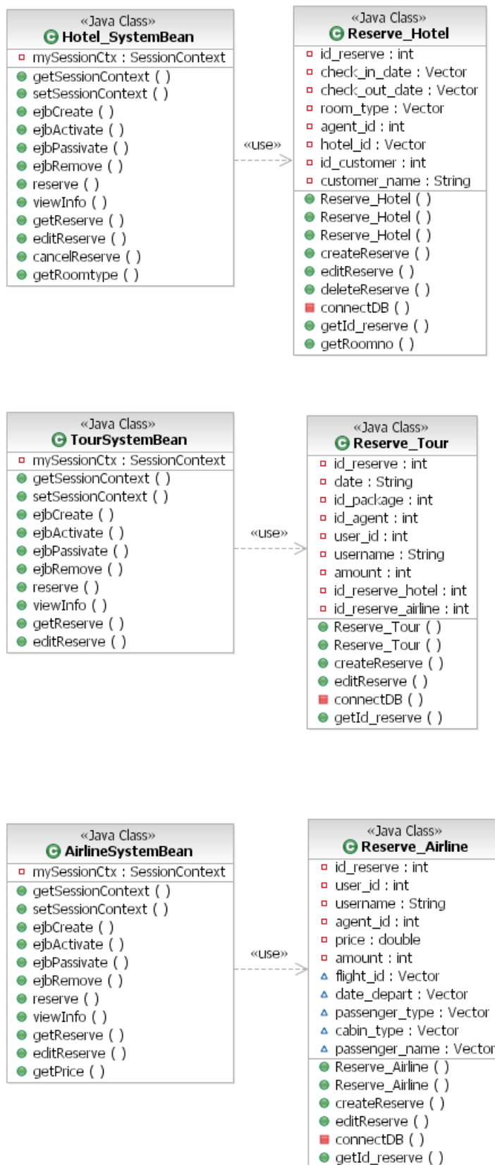
รูปที่ 6.20 Class diagram
