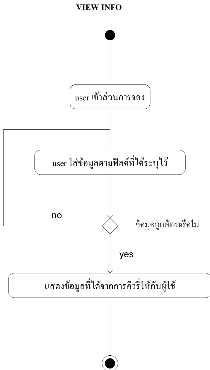
รูปที่ 6.13 Activity diagram (View Info)
