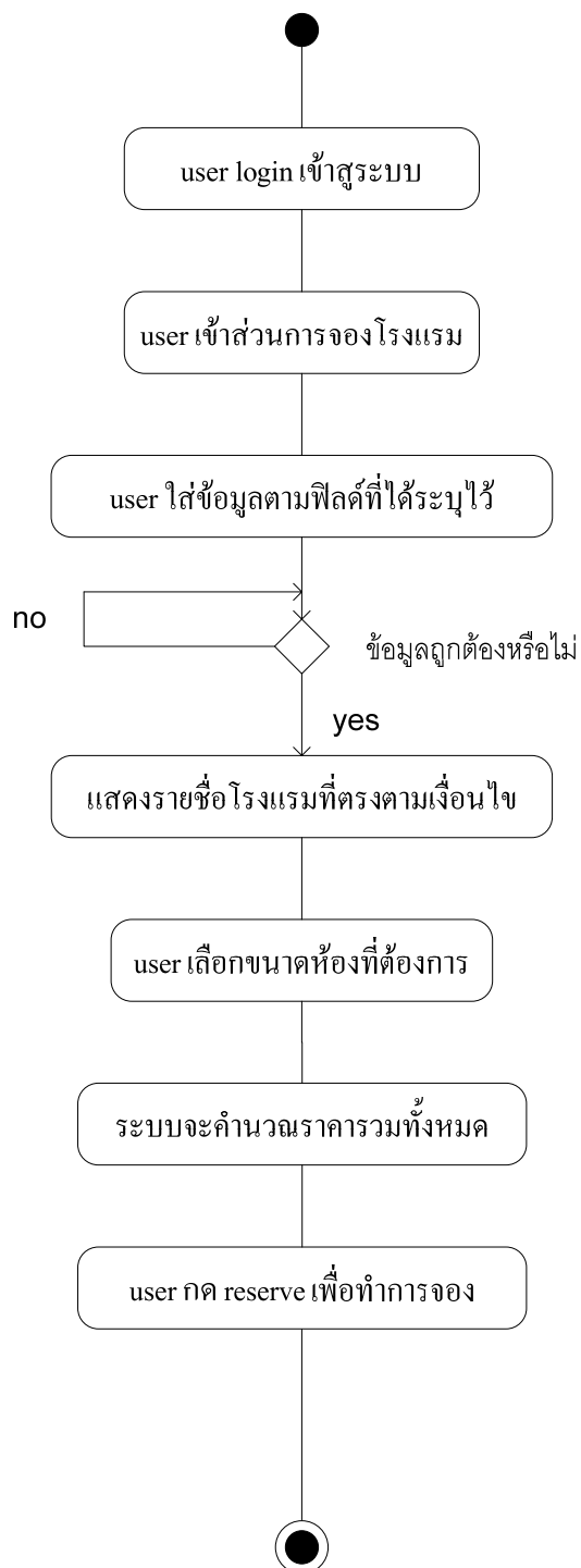
รูปที่ 6.14 Activity diagram (Reserve Hotel)
