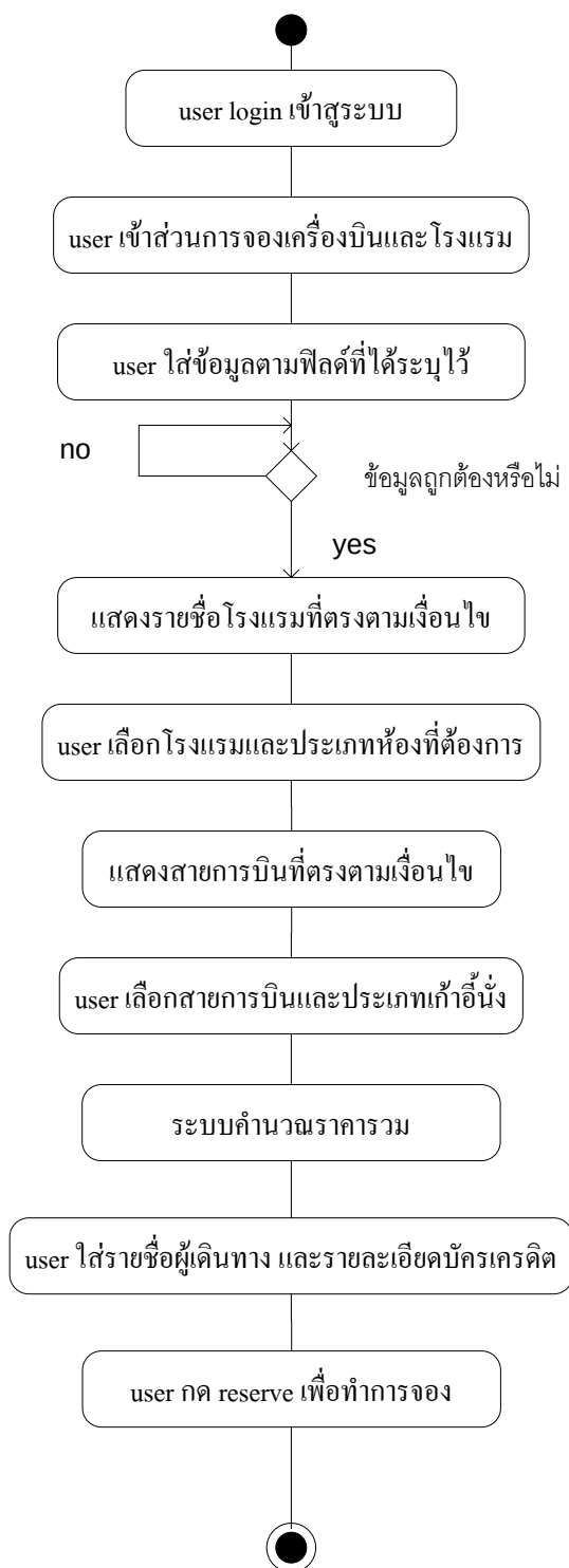
รูปที่ 6.16 Activity diagram (Reserve Hotel_Airline)
