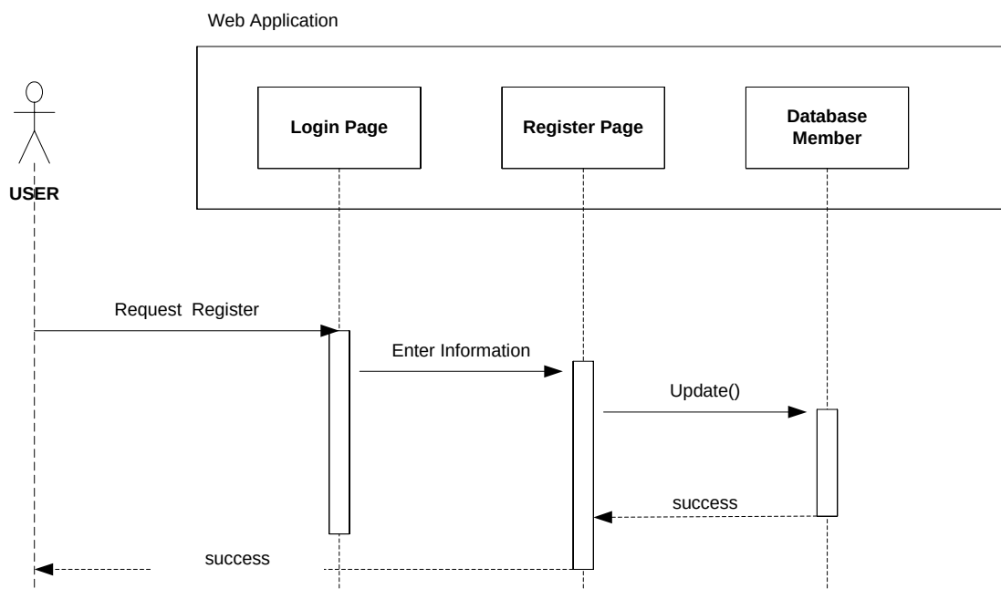
រូបភាព 6.4 Sequence diagram (Register)
