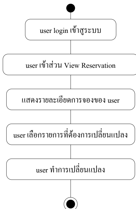
รูปที่ 6.19 Activity diagram (Edit Reservation)
