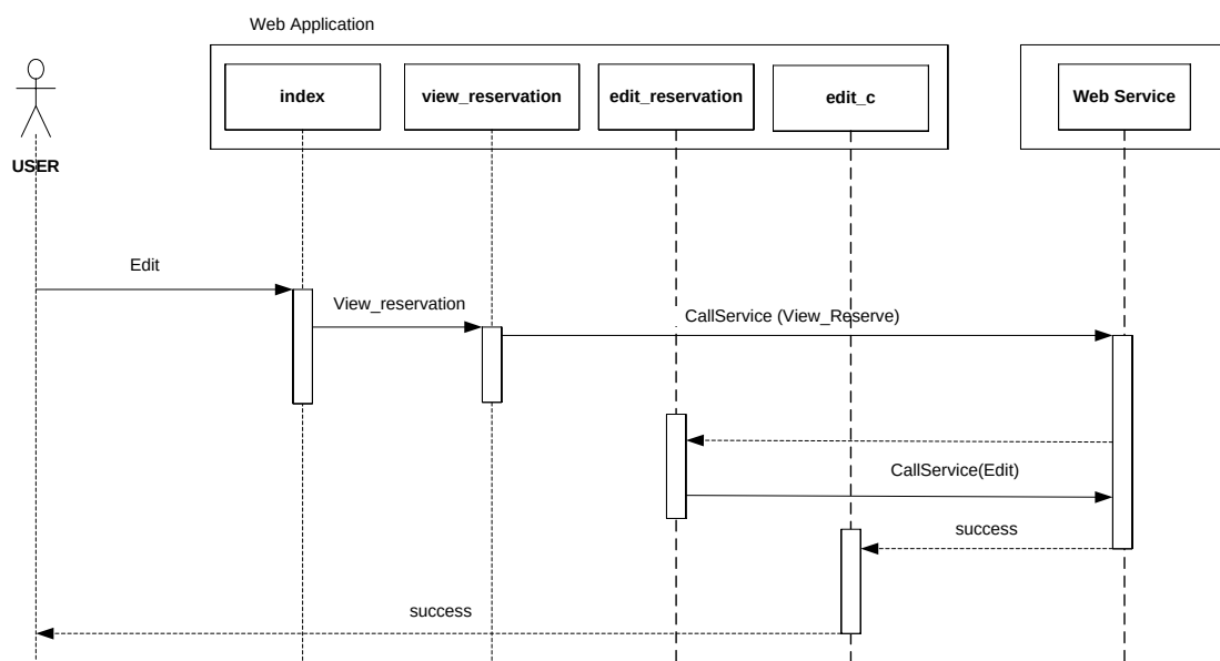
รูปที่ 6.10 แสดง Sequence diagram (Edit)
