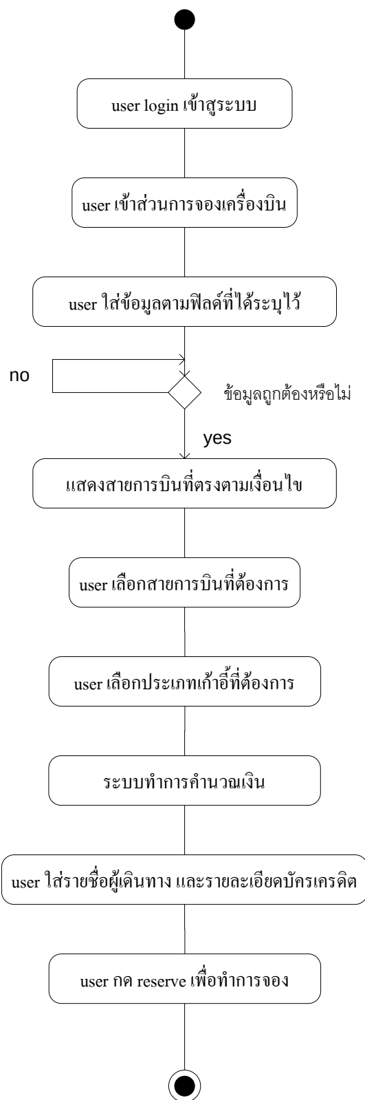
รูปที่ 6.15 Activity diagram (Reserve Airline)
