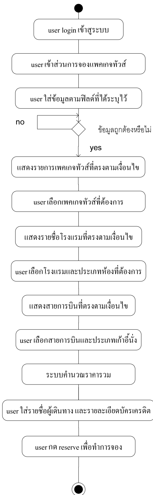
รูปที่ 6.17 Activity diagram (Reserve Package Tour)
