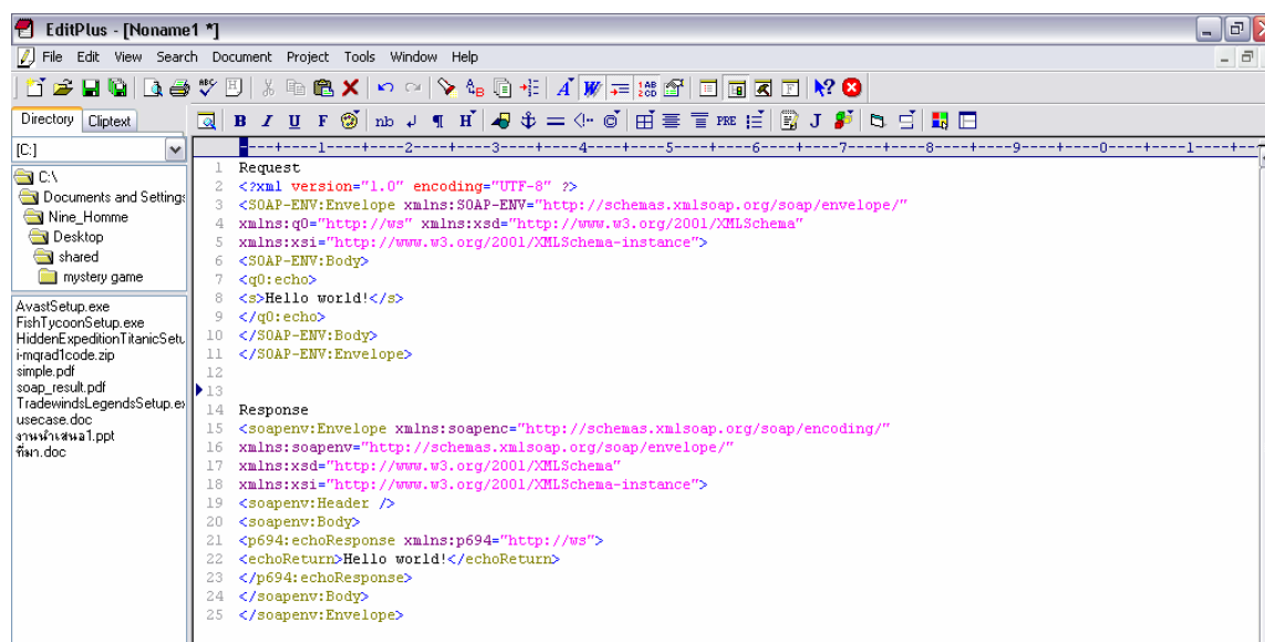
รูปที่ 7.26 SOAP Message ก่อนการทำ WS-security
