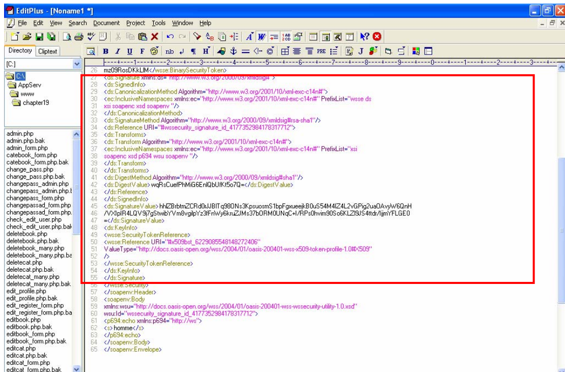
รูปที่ 7.29 SOAP มีการทำ XML Digital Signature
