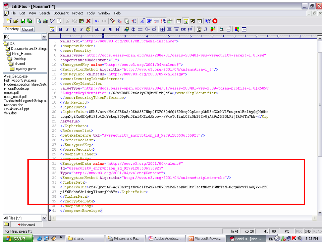
รูปที่ 7.28 SOAP มีการทำ XML Encryption
