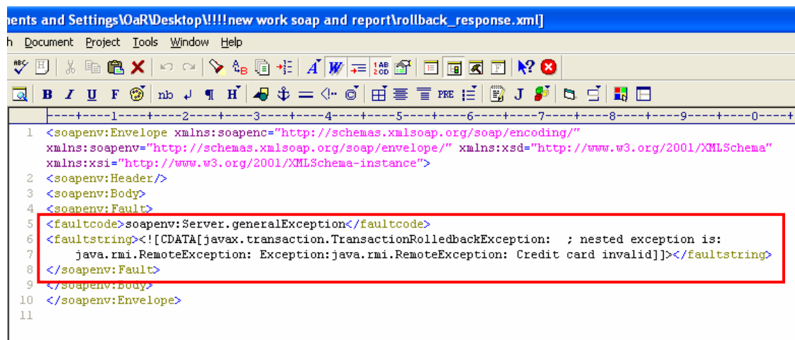
รูปที่ 7.25 SOAP Message ที่มีการระบุว่ามี การ roll back เกิดขึ้น
