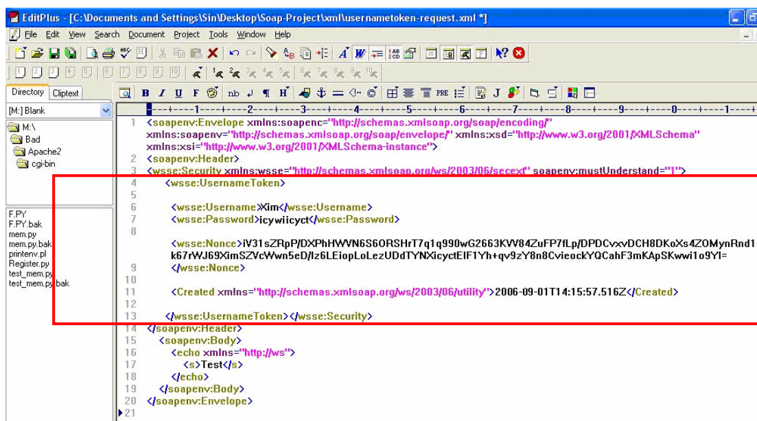
รูปที่ 7.27 SOAP ที่มีการทำ Username Token
