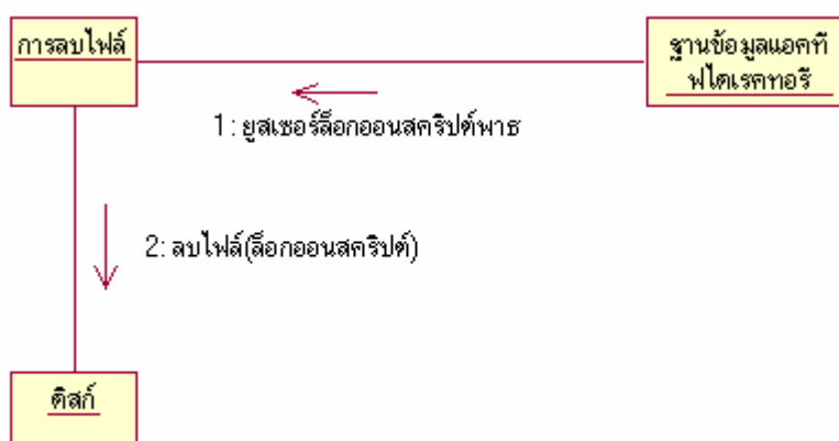
รูปที่ 8.3จ แผนภาพแสดงการทำงานร่วมกันของการลบไลอ้อนสคริปต์
