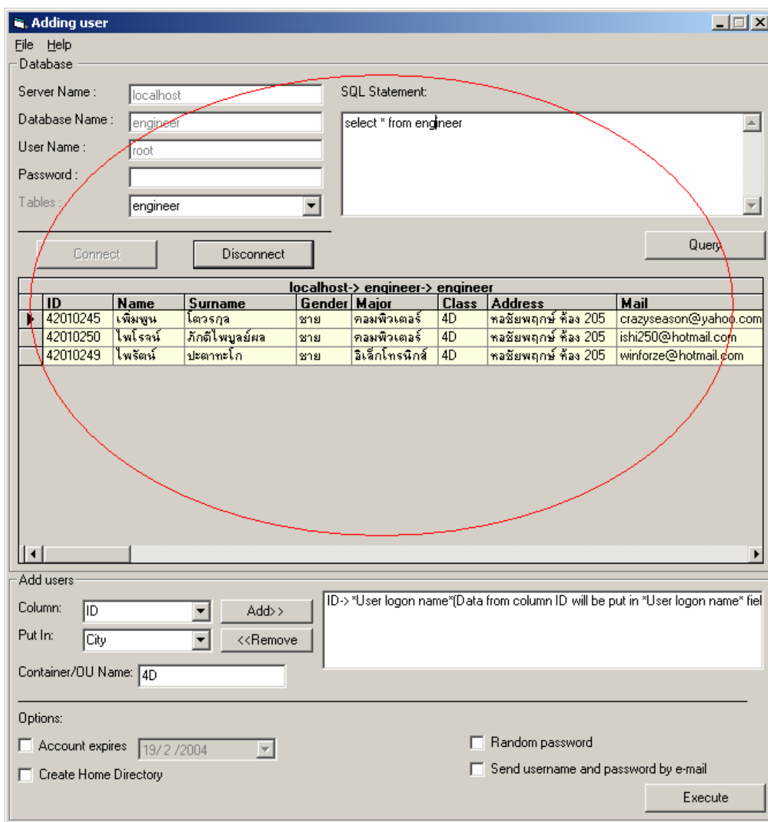
รูปที่ 8.2ก ยูสเซอร์อินเตอร์เฟซที่ใช้ในส่วนของการติดต่อกับฐานข้อมูล
