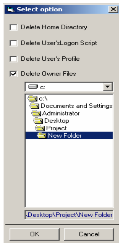
รูปที่ 8.4 ข ยูสเซอร์อินเตอร์เฟซของการการอินพุต ต้องการลบโฮมไดเร็กทอรีหรือไม่, ต้องการลบยูสเซอร์โฟลเดอร์หรือไม่, ต้องการลบสคริปต์หรือไม่ว่าไดเร็กทอรีที่ต้องการหาไอคอนไฟล์
