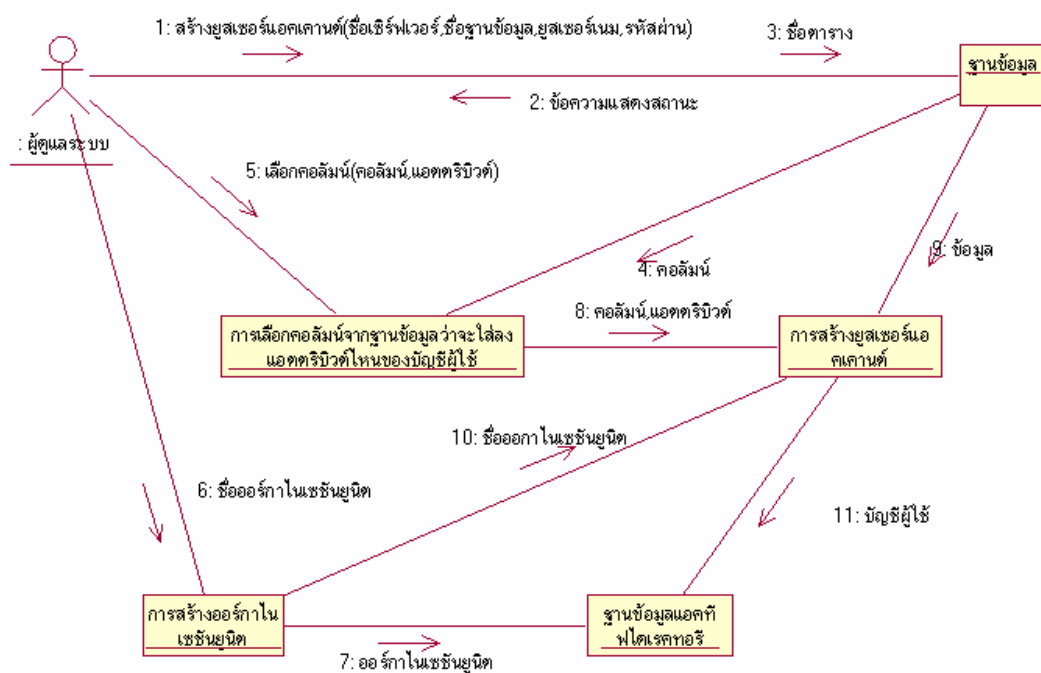
รูปที่ 8.1x แผนภาพแสดงการทำงานร่วมกันของการสร้างบัญชีผู้ใช้งาน
