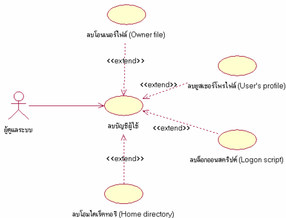
รูปที่ 8.3ก แสดงยูสเคสการออกแบบเครื่องลบบัญชีผู้ใช้
