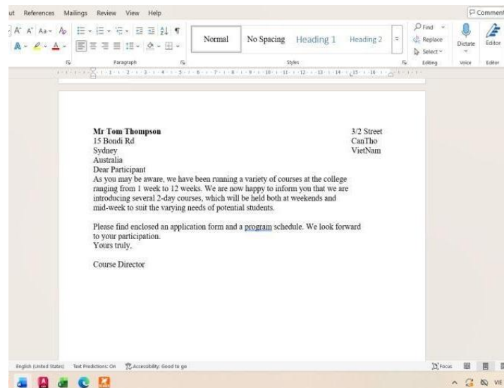
Hình 2-1 Văn bản mẫu thư mời thực hiện trên Microsoft Word
